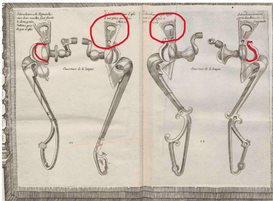
Obr. 16 – Oko pro upevnění licnic (Pluvinel 1666).
