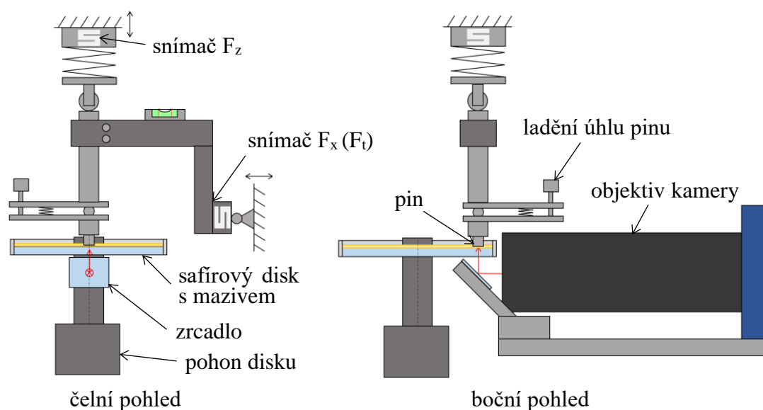
Obr. 4-2 Schéma měřicí soustavy tribometru a kamery
