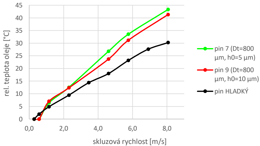
Obr. 5-35 Porovnání teplot oleje – pin 7, pin 9 a hladký pin – paralelní povrchy (50 N)
