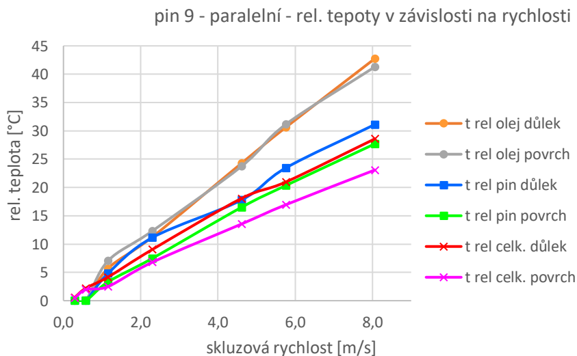
Obr. 5-31 Celkové rel. teploty a rel. teploty pinu a oleje v kontaktu – pin 9 paralelní povrchy (50 N, h_0=10 \mu\text{m} )
