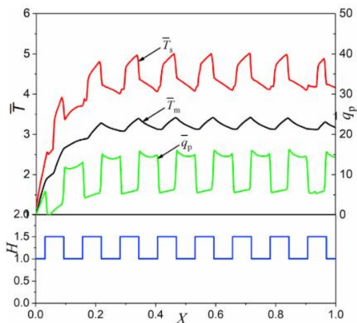
Obr. 2-16 Teplota a lokální tepelný tok na střednici ( T_s je teplota slideru, T_m je teplota maziva a q_p je lokální tepelný tok do hladké desky) [22]
