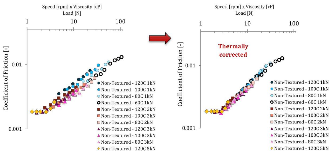
Obr. 2-5 Korekce Stribeckovy křivky vzhledem k znalosti teploty v kontaktu [8]
