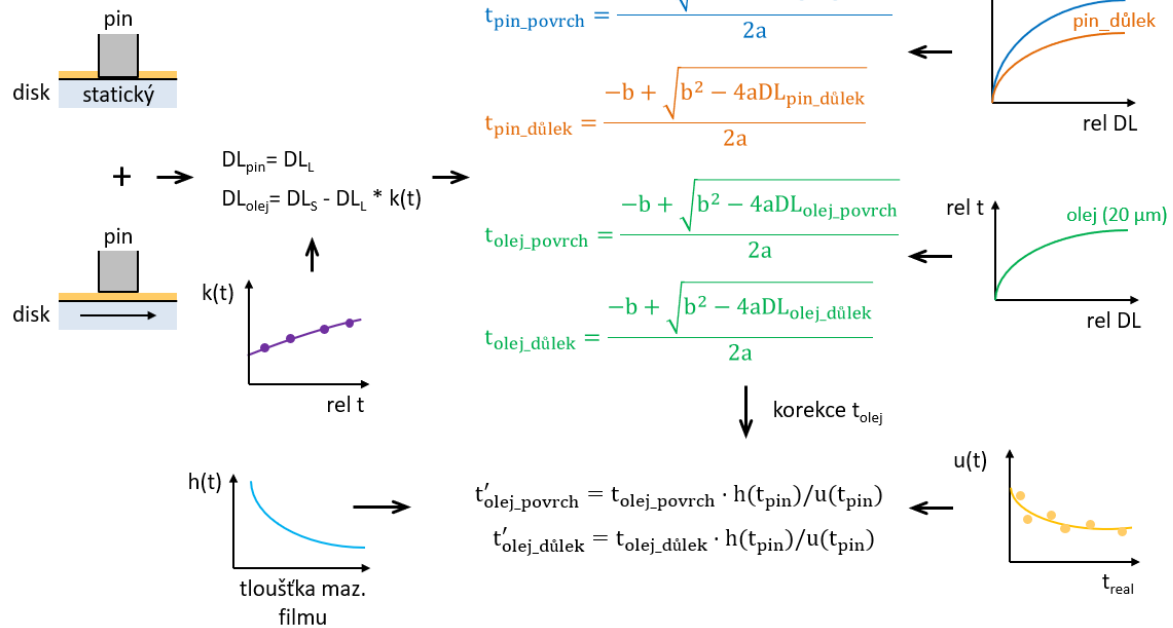
Obr. 5-16 Schéma postupu měření a vyhodnocení teploty texturovaných pinů a oleje
