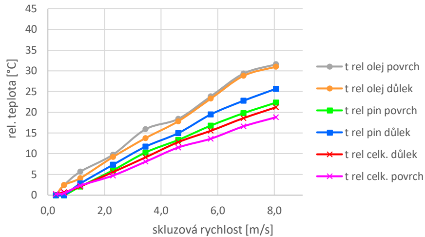
pin 7 - klínová spára - rel. teploty v závislosti na rychlosti
