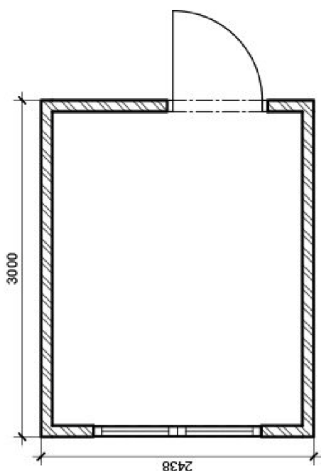
Obrázek [9]: Půdorys BK2
