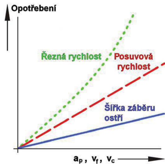
Obr. 7 Závislost celkového opotřebení na řezných podmínkách [5]
