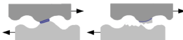
Obr. 10 Princip adhezního opotřebení [39]
