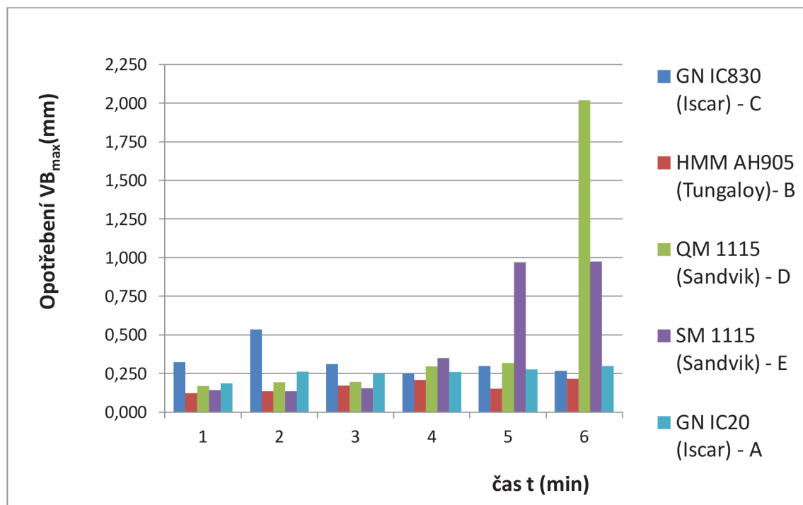
Obr. 14 Závislost opotřebení VB_{max} na čase u jednotlivých typů VBD
