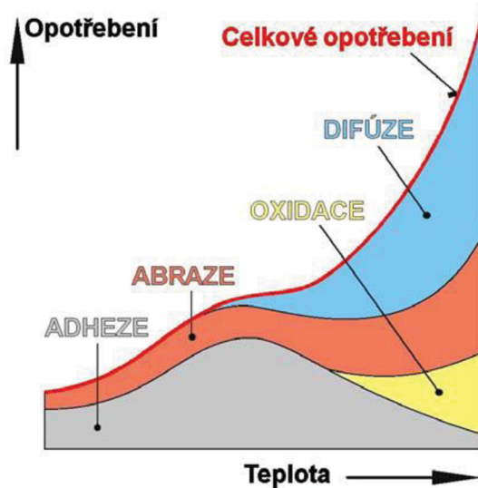
Obr. 6 Vliv teploty na aktivitu jednotlivých mechanismů opotřebení [5]
