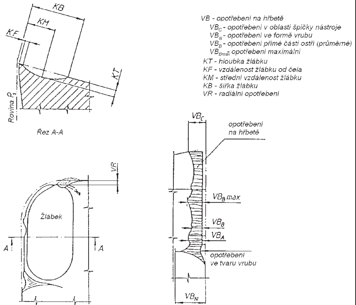
Obr. 13 Klasifikace opotřebení břitu nástroje dle ISO 3685 [44]
