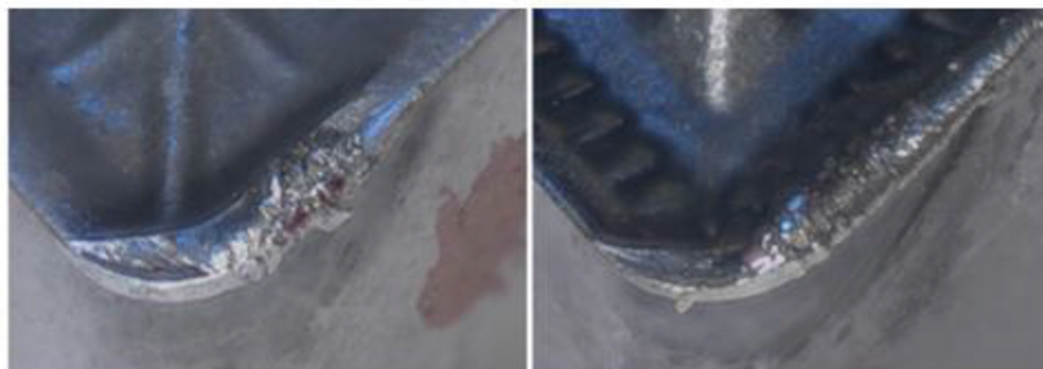
Obr. 17 Srovnání opotřebení čela VBD
