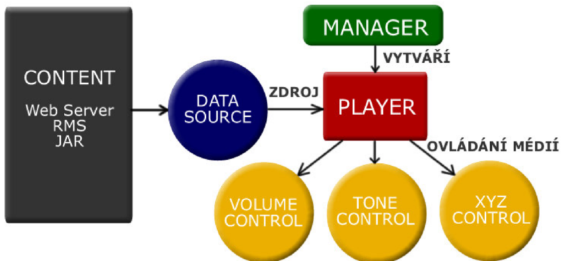
Obr. 5: Architektura MMAPI
