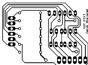
Obr. 2.5: Návrh DPS pro negátory výstupu IR čidel
