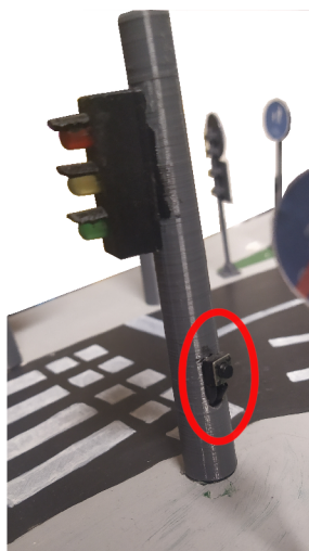
Obr. 2.1: Umístění mikrospínače pro nastavení požadavku překonání komunikace
