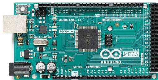
Obr. 2.12: Arduino Mega 2560 [5]
