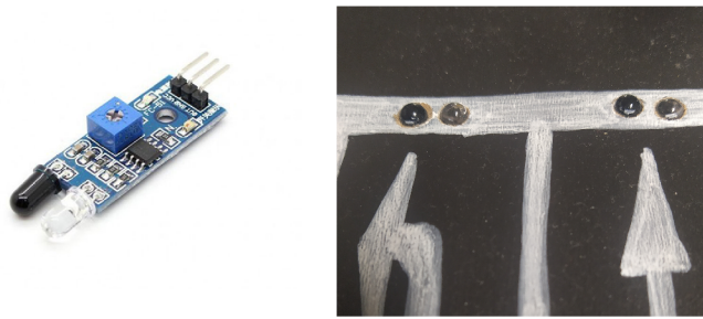
Obr. 2.13: IR senzor [7] a jeho instalace
