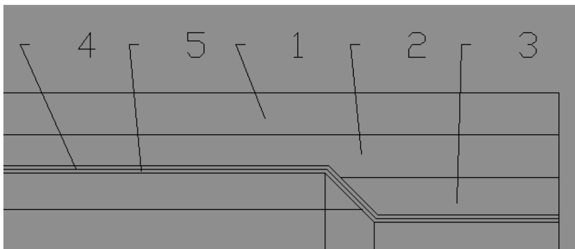
Obr. 3.18 – Závit M80x4.
