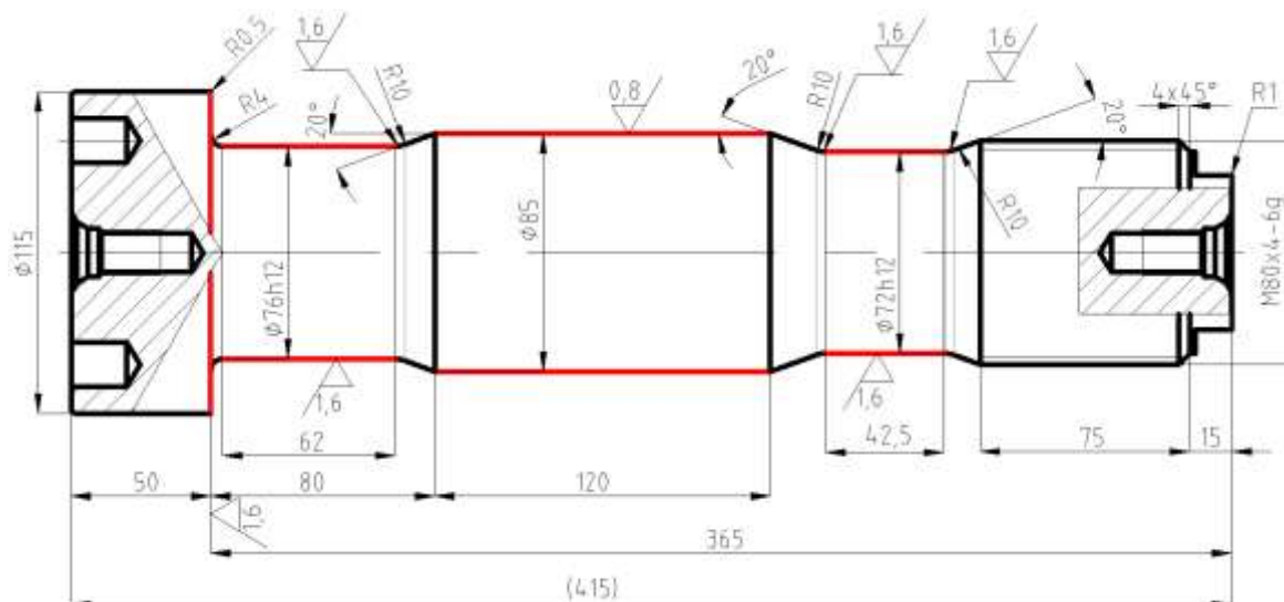
Obr. 3.7 – Náčrt součásti.
