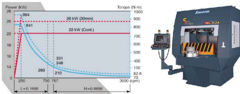
Obr. 2.5 – Příklad obráběcího centra VTC-650 + Charakteristika výkonu [14].
