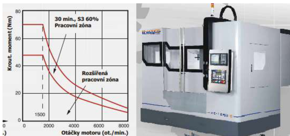
Obr. 2.6 – Příklad obráběcího centra INAXES + charakteristika kroučícího momentu [15].
