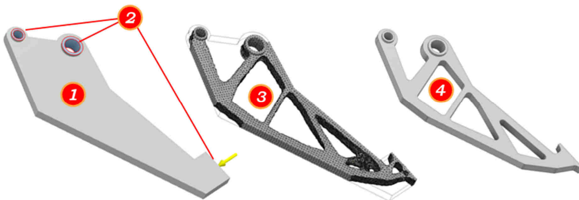
Obr. 38 Autodesk Inventor 2016 R2 - Generátor tvarů [23]
