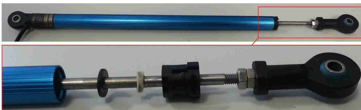
Obr. 29 Lineární potenciometrický snímač polohy Penny & Giles SLS 130/75/L/50
