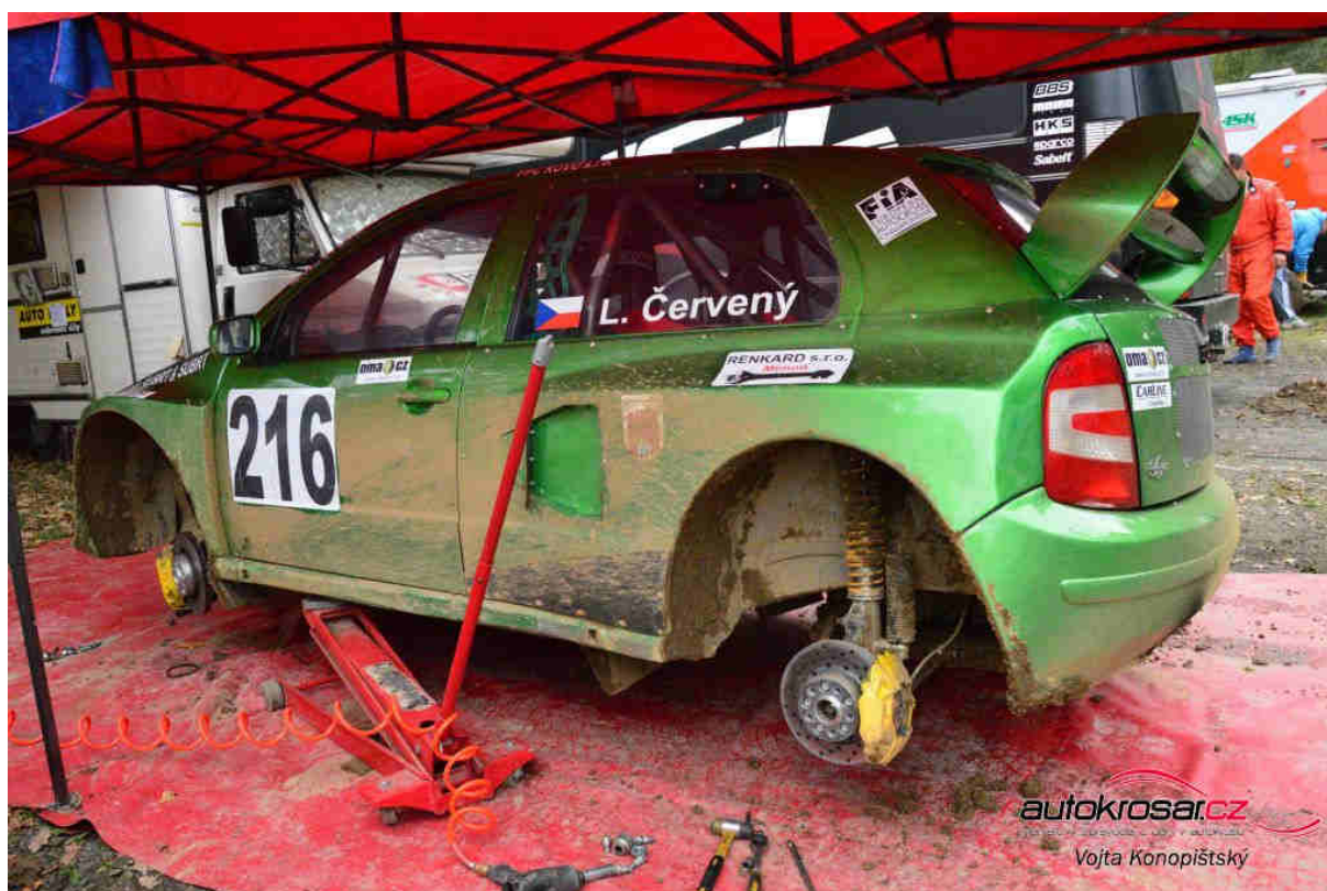
Obr. 3 Pohled na zavěšení MacPherson autokrosového vozidla [6]
