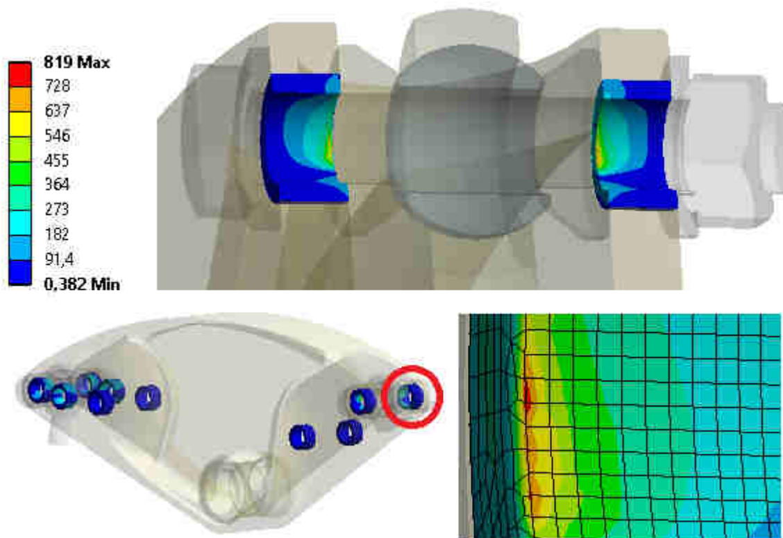
Obr. 66 První vývojová verze se šrouby M12, oc. vložkami – ekvivalentní napětí ocelových vložek [MPa]
