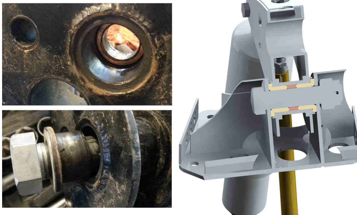
Obr. 26 Uložení vahadla kluznými ložisky - vlevo reálné součásti, vpravo model sestavy
