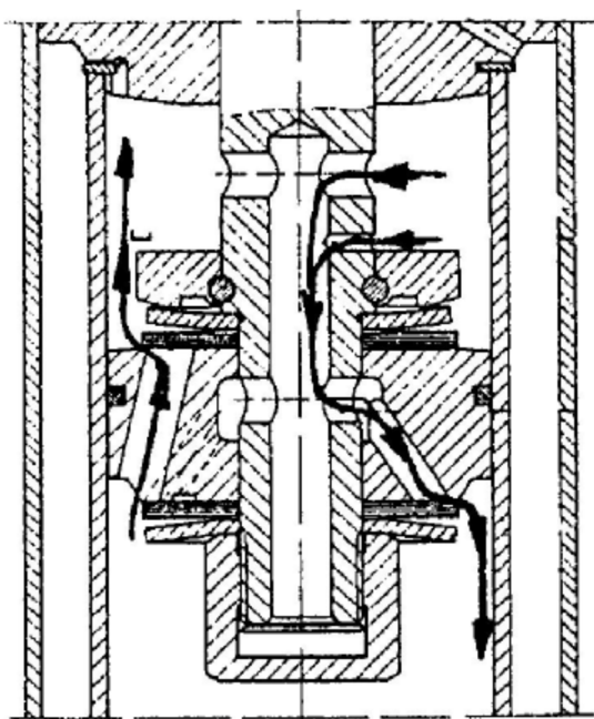
Obr. 9 Příklad řešení dolního hydraulického dorazu [2]
