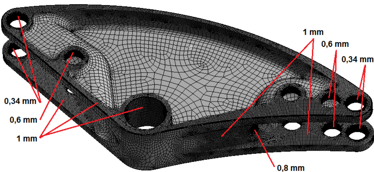
Obr. 79 Pohled sítě výsledného konstrukčního řešení vahadla
