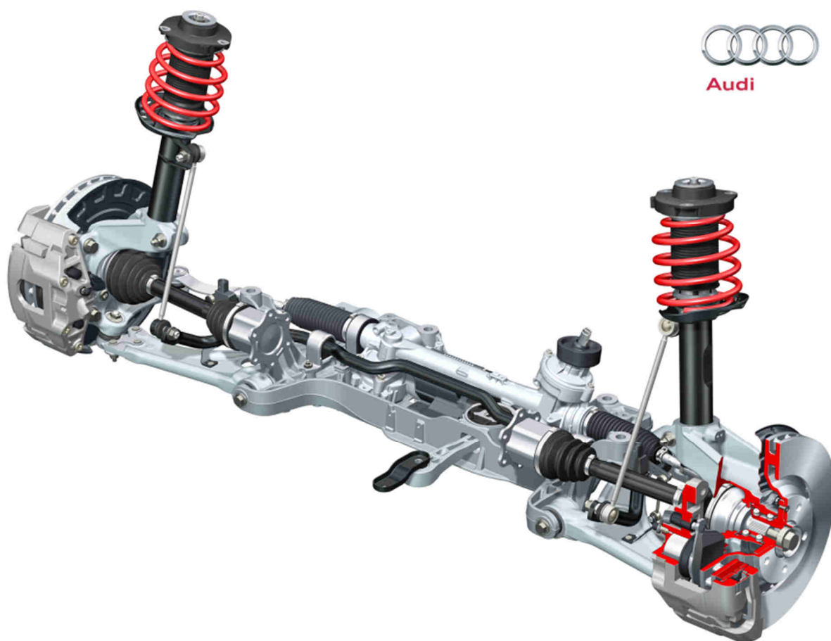
Obr. 2 MacPherson přední poháněná náprava Audi TT [5]
