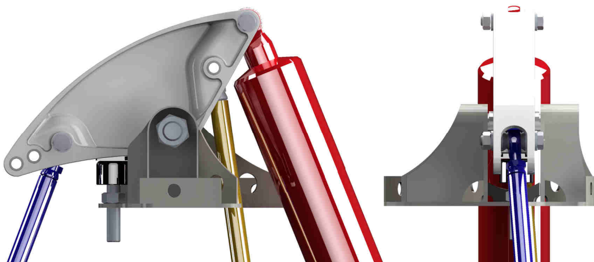
Obr. 93 Detailní pohled modelu vahadla a navazujících prvků výsledného konstrukčního řešení
