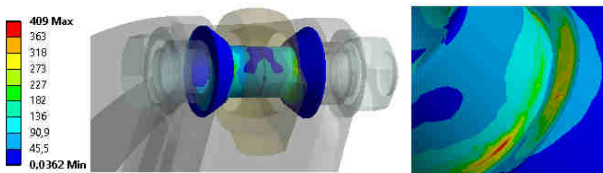
Obr. 86 Výsledné konstrukční řešení – ekvivalentní napětí vymežovacích vložek [MPa]
