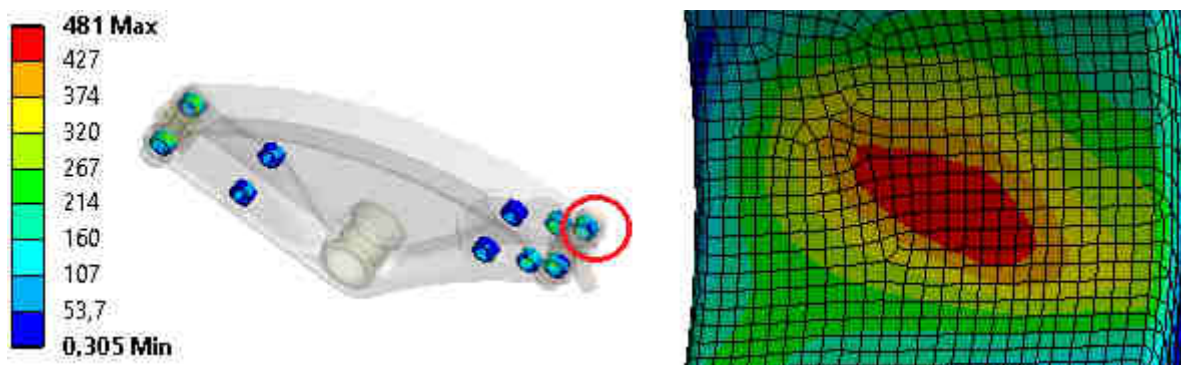
Obr. 87 Výsledné konstrukční řešení – ekvivalentní napětí ocelových vložek s radiusem [MPa]
