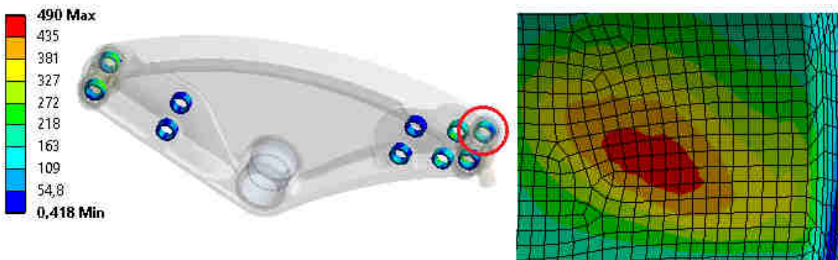
Obr. 75 Druhá vývojová verze – ekvivalentní napětí ocelových vložek s radiusem [MPa]
