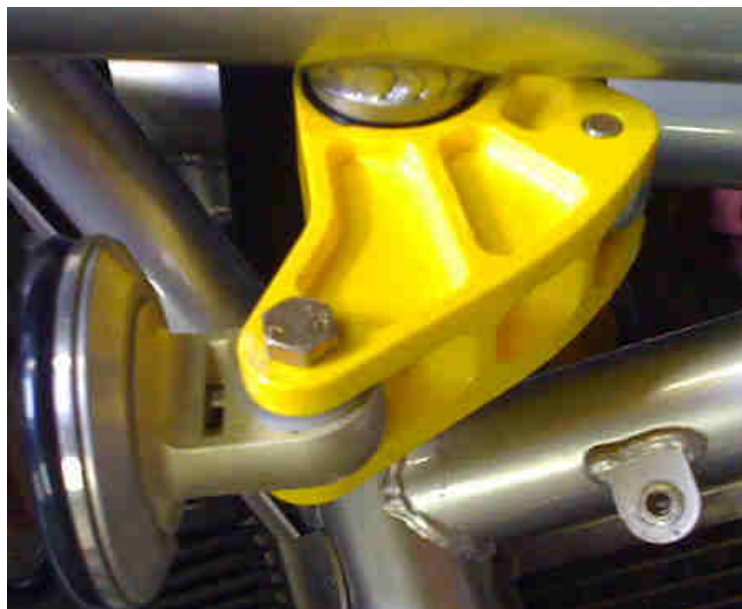
Obr. 18 Ariel Atom - náhrada originálního vahadla plastovým prototypem [16]
