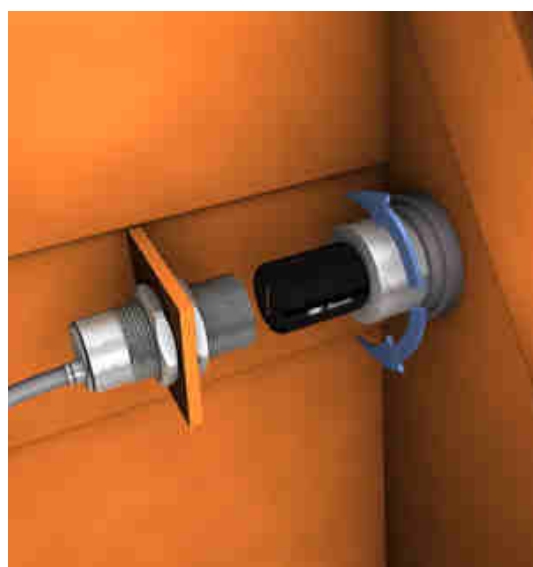
Obr. 31 Magnetický snímač měření úhlu [28]
