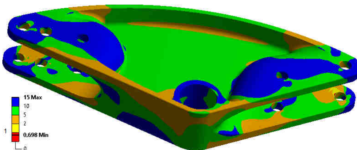
Obr. 54 První vývojová verze se šrouby M12 – koeficient bezpečnosti vůči meznímu stavu pružnosti
