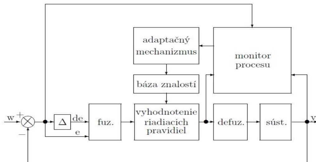
Obrázok 17: Bloková schéma adaptívneho fuzzy regulátora [13]
