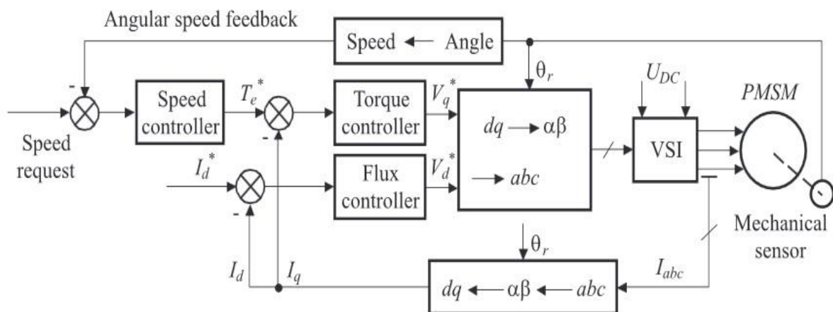
Obrázok 13: Blokové schéma vektorového riadenia [1]
