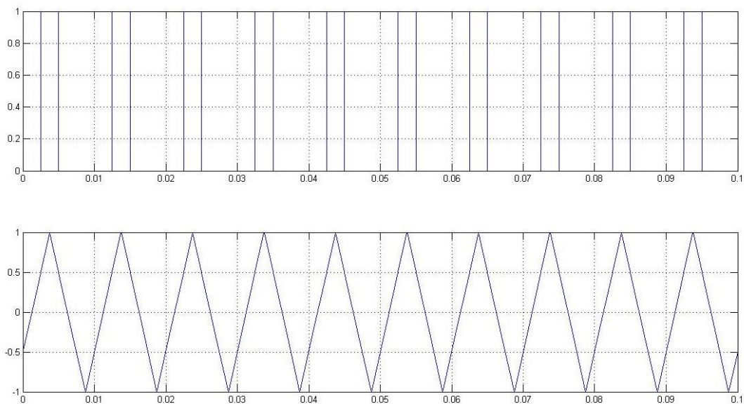
Obrázok 6: PWM signál
