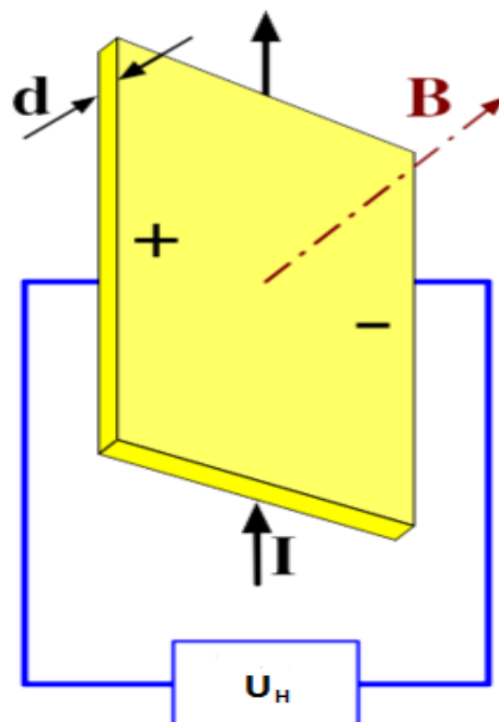
Obrázok 10: Hallov jav
