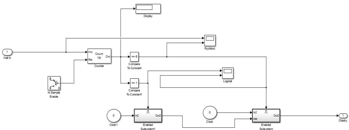
Obrázok 29: Interpolácia -1.metóda
