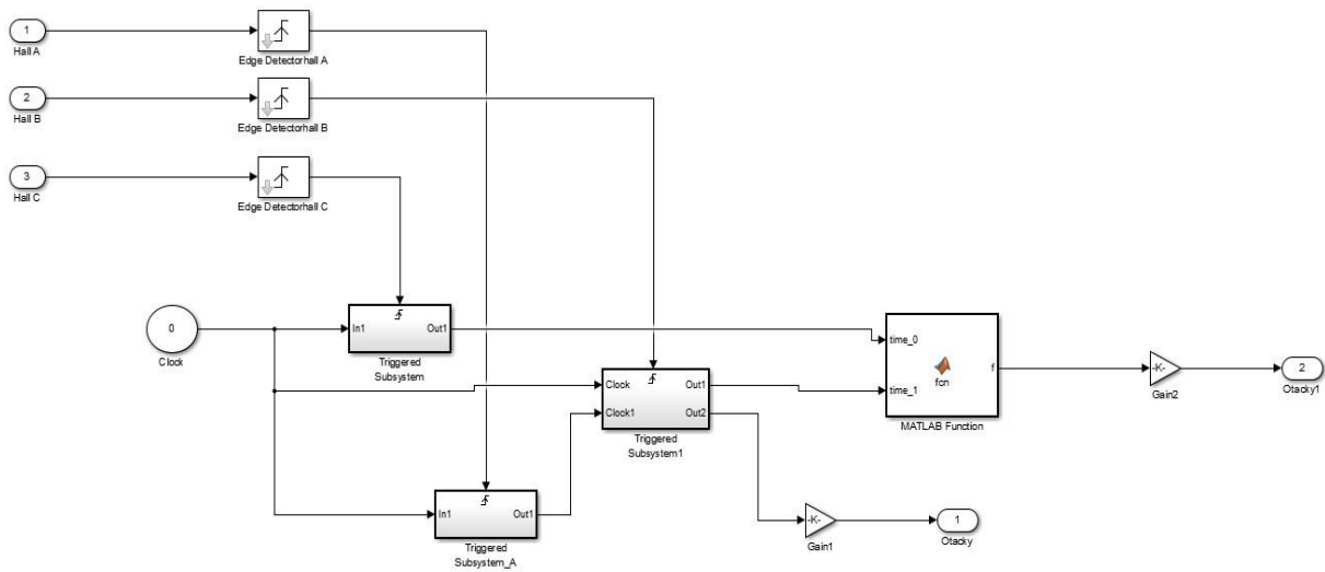
Obrázok 30: Interpolácia – 2.metóda
