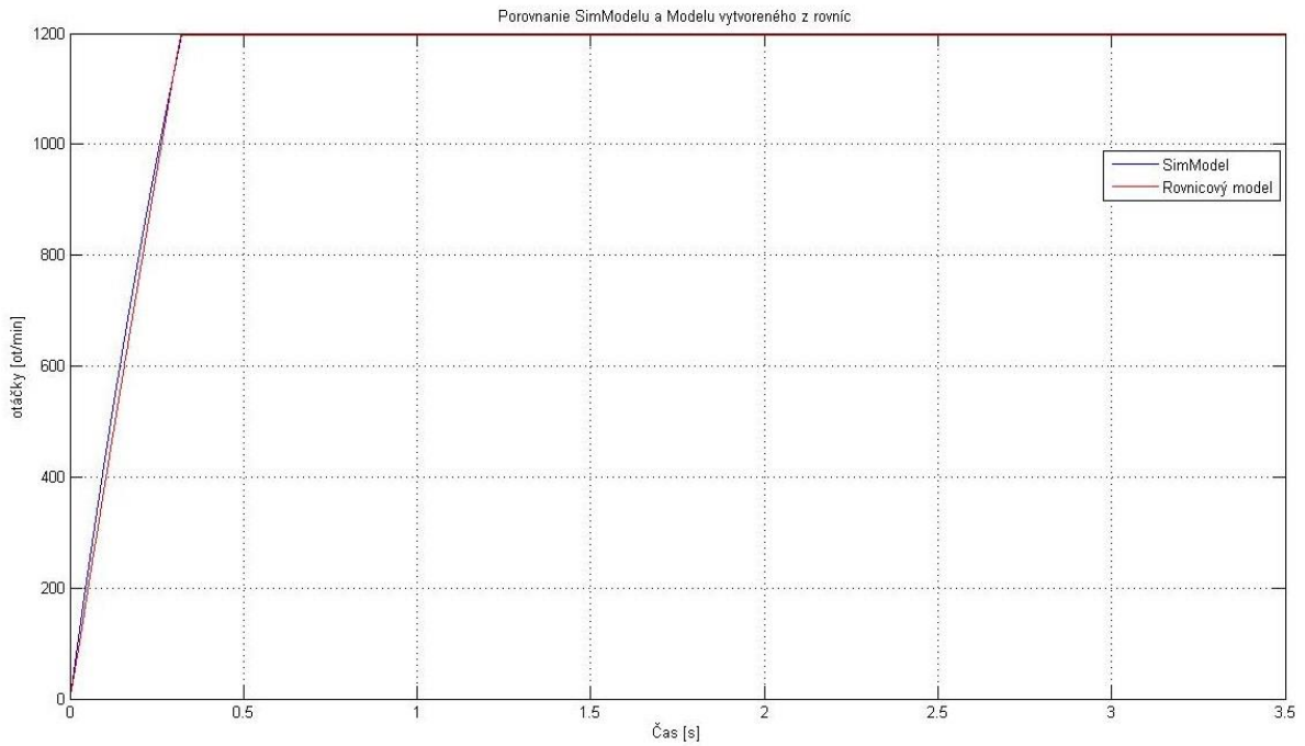
Obrázok 23: Porovnanie prechodových charakteristik
