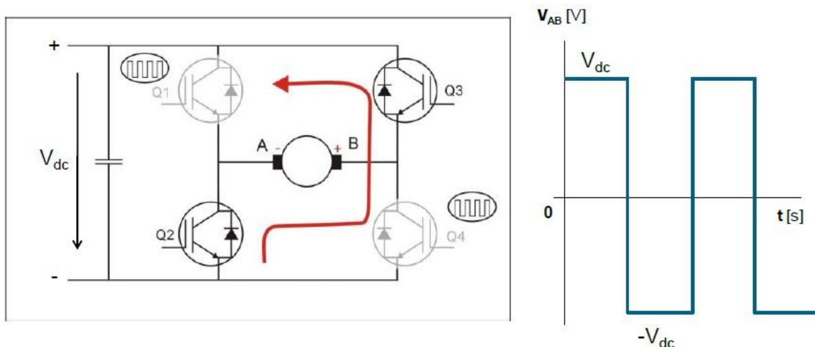
Obrázok 5: Bipolárne spínanie [5]
