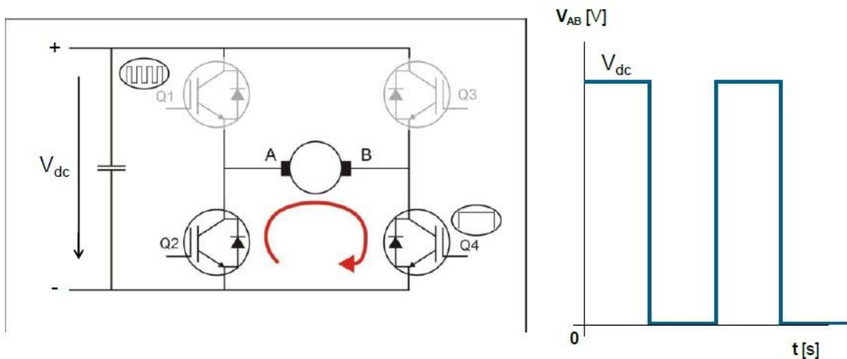
Obrázok 4: Unipolárne spínanie [5]
