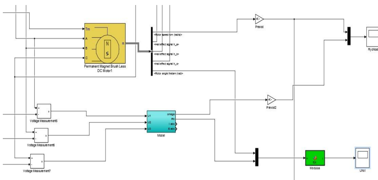
Obrázok 36: Model s matematickým modelom
