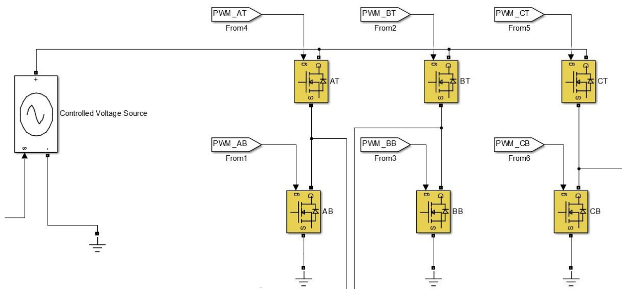
Obrázok 18: Napájacia časť
