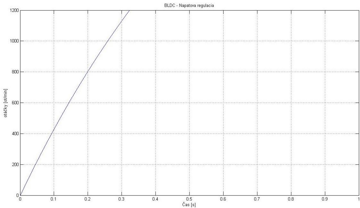
Obrázok 21: Prechodová charakteristika
