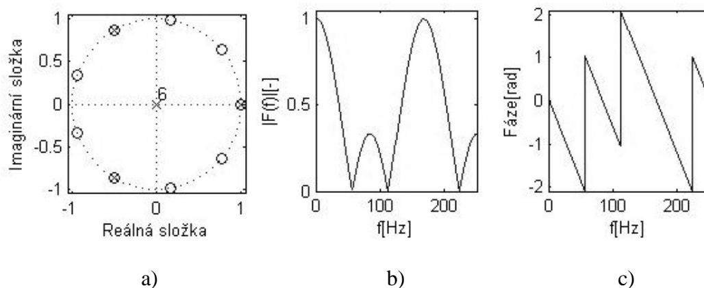
Obr. 5.5 a) Rozložení nulových bodů a pólů na jednotkové kružnici; b), c) amplitudová a fázová charakteristika Lymnovy pásmové propusti 1. typu
