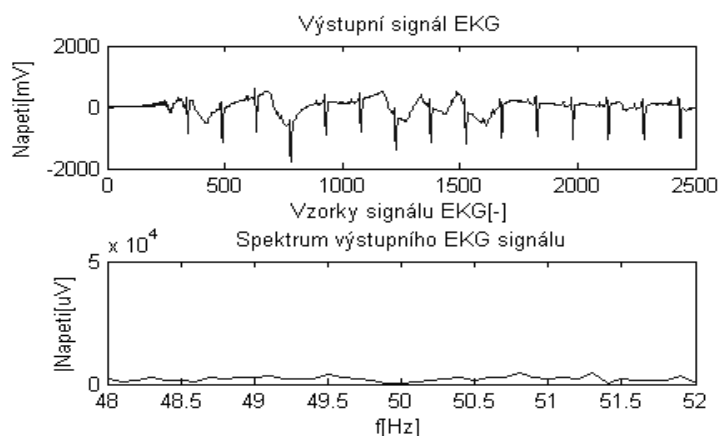
Obr. 7.20 Výstupní signál filtrovaný Lymnovou pásmovou zádrží s šířkou pásma 1 Hz (detail v okolí 50 Hz)
