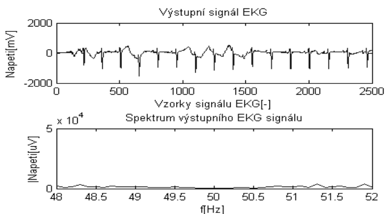
Obr. 7.21 Výstupní signál filtrovaný Lymnovou pásmovou zádrží s šířkou pásma 2 Hz (detail v okolí 50 Hz)
