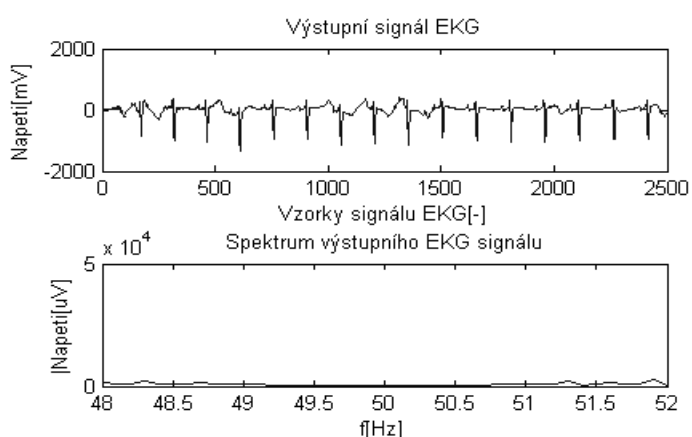
Obr. 7.22 Výstupní signál filtrovaný Lymnovou pásmovou zádrží s šířkou pásma 3 Hz (detail v okolí 50 Hz)
