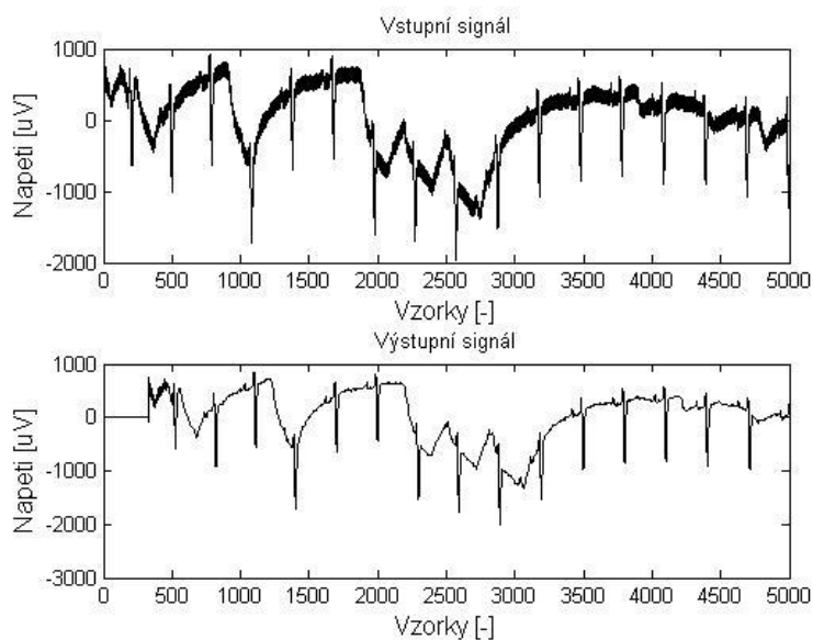
Obr. 6.18 Výsledek filtrace Lymnovou pásmovou zadržkí 2.typu
