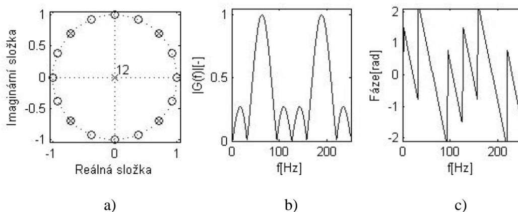
Obr. 5.6 a) Rozložení nulových bodů a pólů na jednotkové kružnici; b), c) amplitudová a fázová charakteristik Lymnovy pásmové propusti 2. typu
