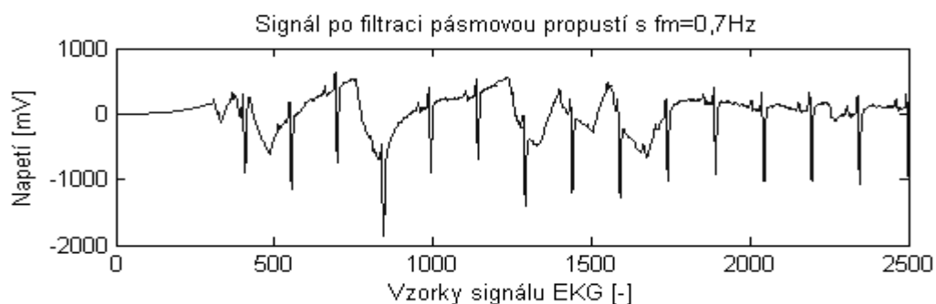
Obr. 7.6 Signál EKG po filtraci horní propustí s mezním kmitočtem f_M = 0,7 \text{ Hz}
