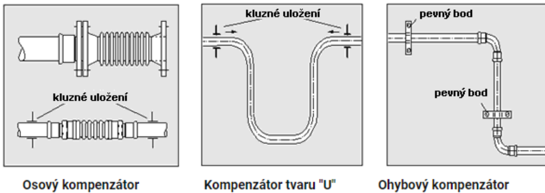
Obrázek 7 - Druhy kompenzátorů [18]
