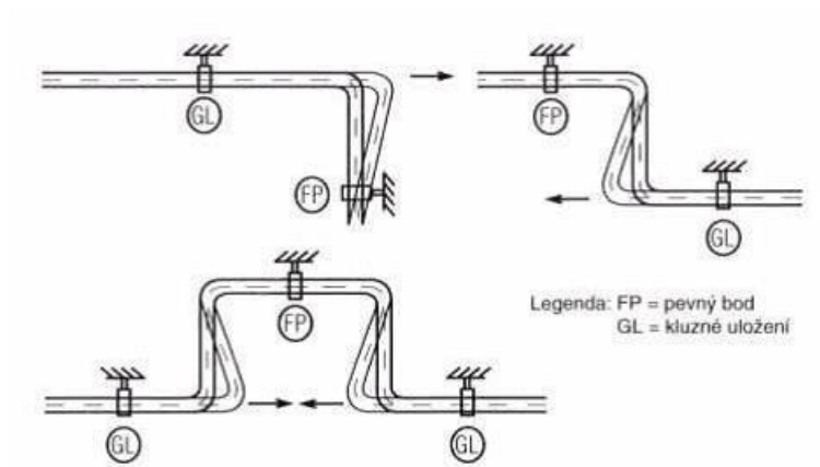
Obrázek 8 - Příklady řešení kompenzaci ohybem [19]
