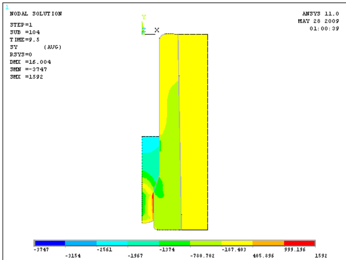
Obr. 34 Osová napětí při redukci 56 %
