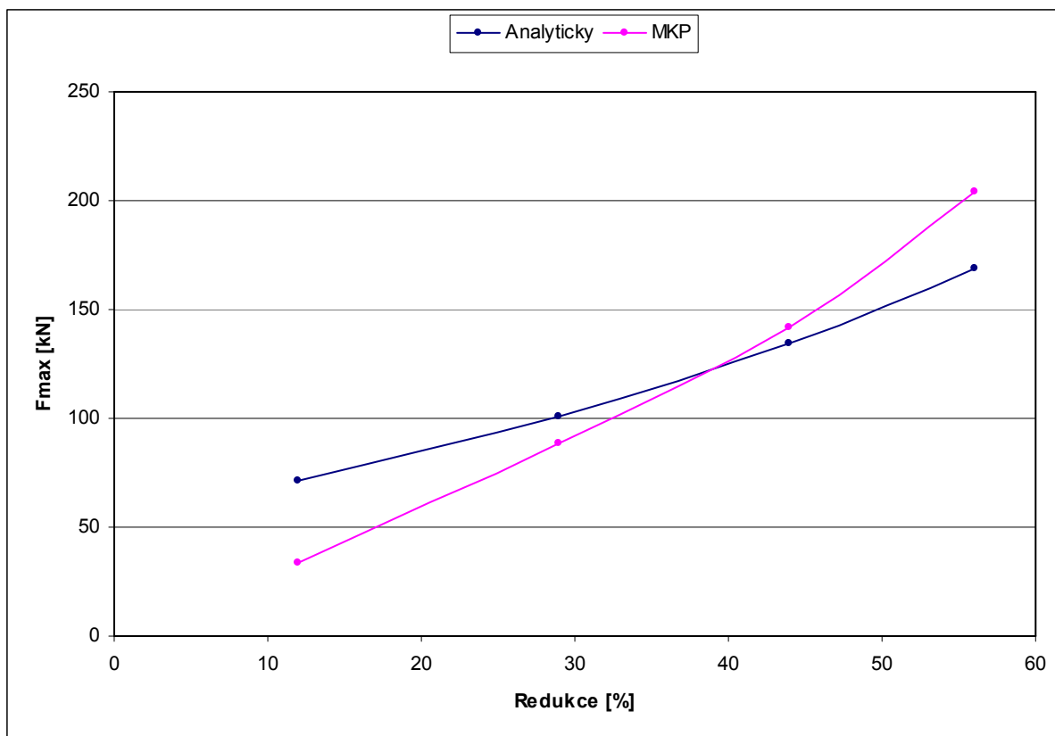
Obr. 15 Maximální protlačovací síla v závislosti na redukcí.
