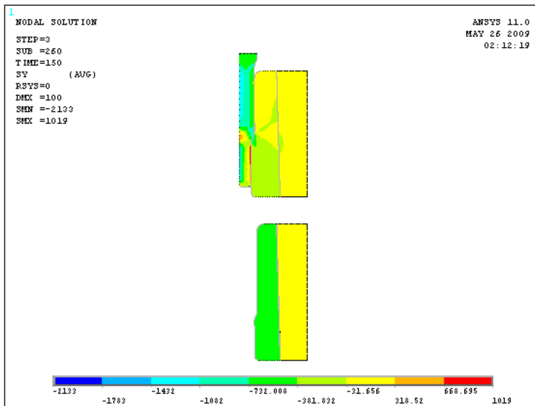
Obr. 37 Osová napětí po 2. kroku protlačování
