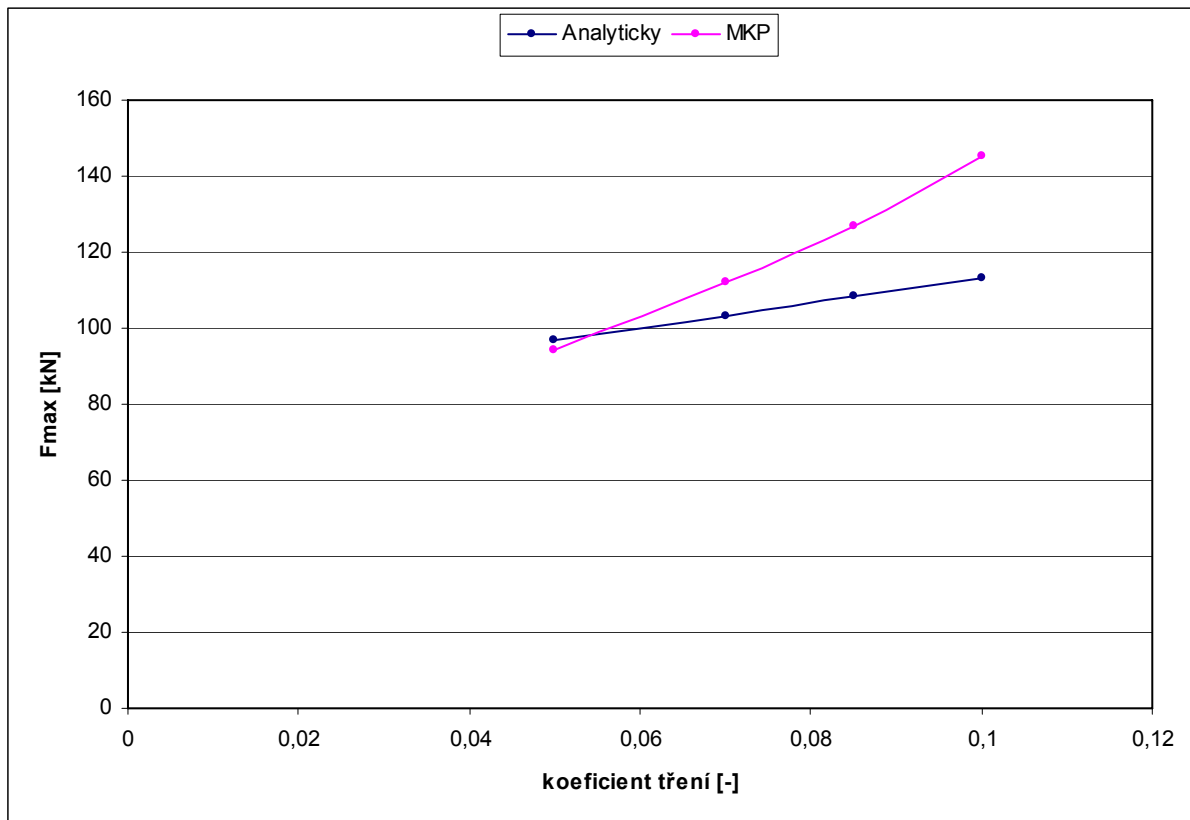
Obr. 21 Vliv koeficientu tření na maximální protlačovací sílu
