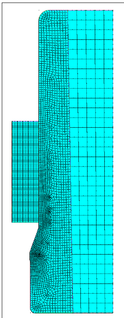
Obr. 7 Síť MKP
