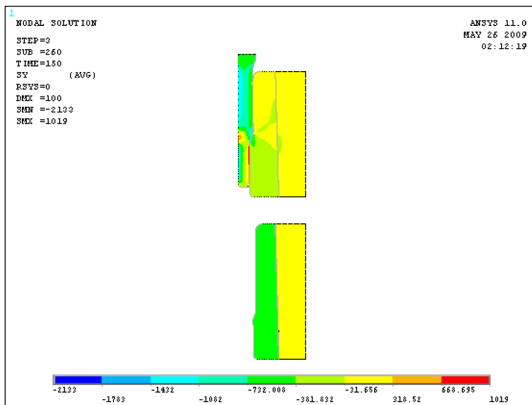
Obr. 37 Osové napětí po 2. kroku protlačování
