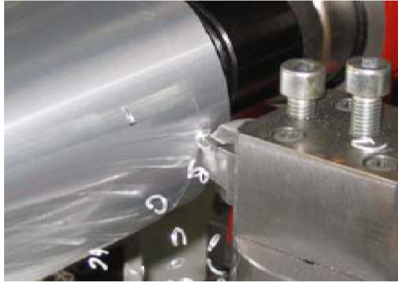
Obr. 3.3 Tvorba krátké člankovité třísky (9)
