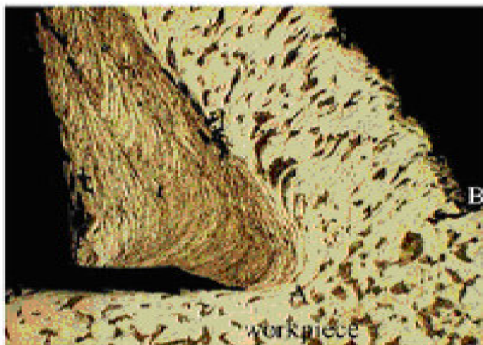
Obr. 4.1 Vznik adheze (9)
