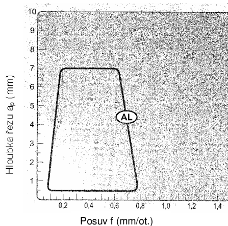
Obr. 4.4 Funkční diagram (5)
