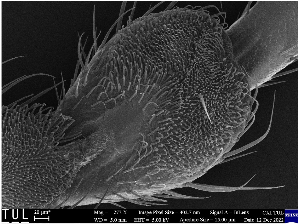
Obr. 28: SEM - pulvilli
