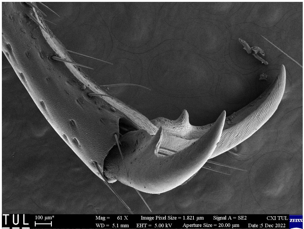
Obr. 51: SEM - drápy
