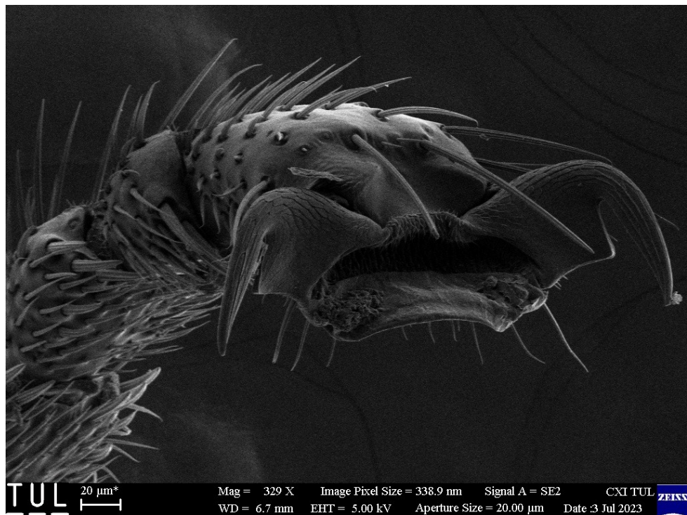
Obr. 61: SEM - drápy
