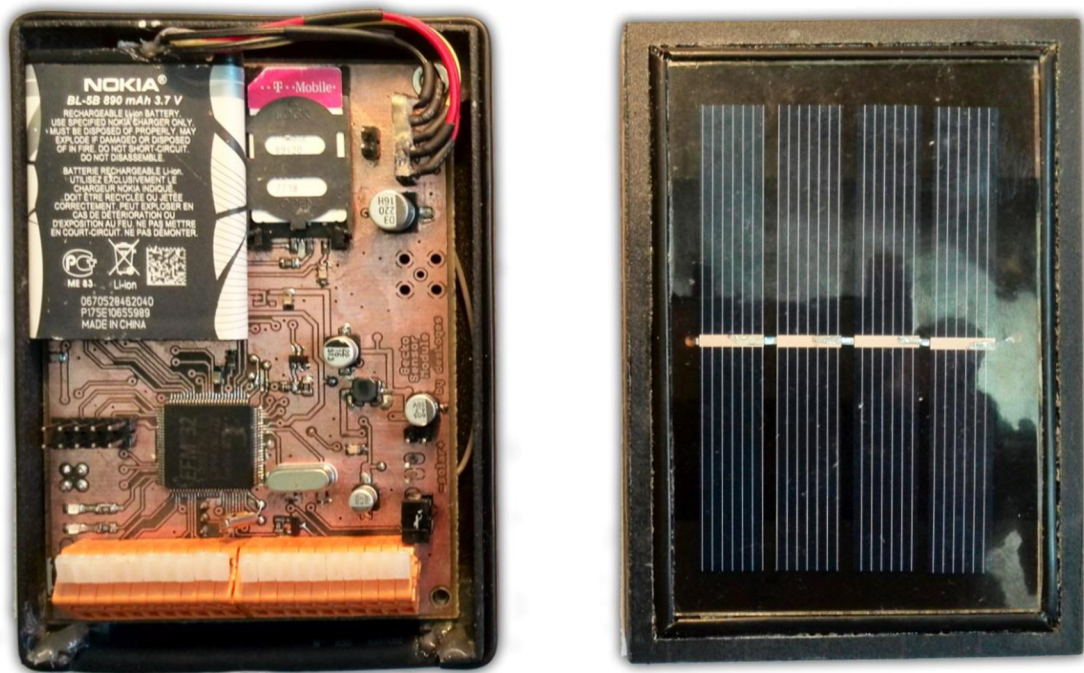
Obr. 5-22 Hotový nízkoenergetický senzorový modul - otvorený
