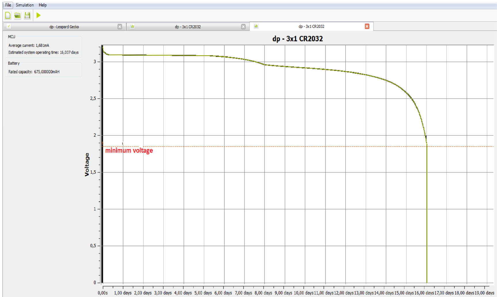
Obr. 5-15 Simulácia výdrži akumulátora pomocou softvéru eBattery
