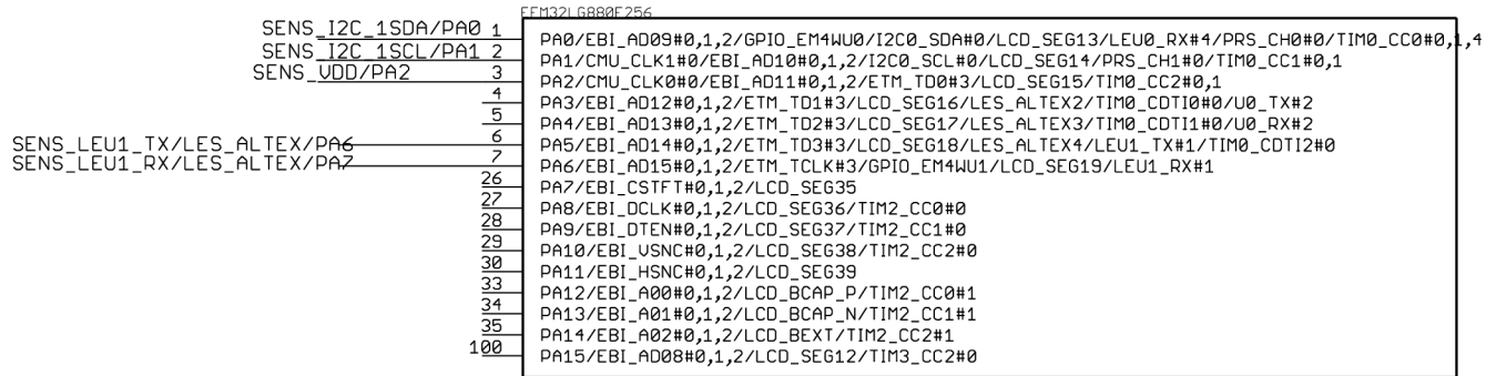
Obr. 5-2 Schéma zapojenia EFM32L G880F256 mikrokontroléru (časť 1.)
