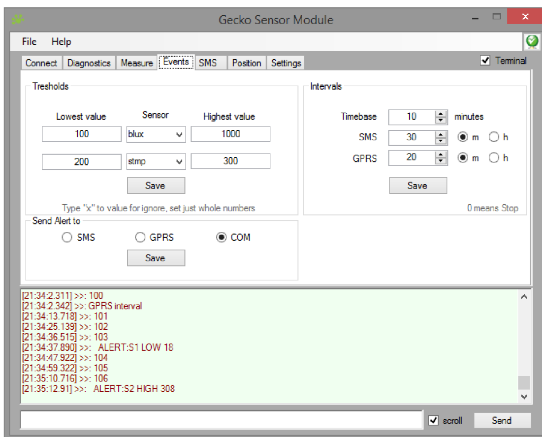
Obr. 4-11. GUI - udalosti
