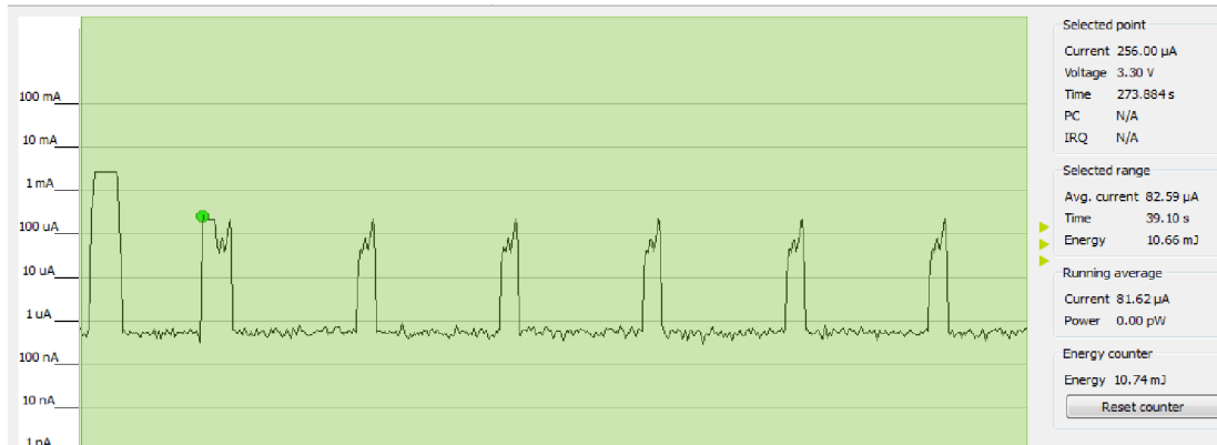
Obr. 4-20 Meranie spotreby - senzory sú napájané zvlášť
