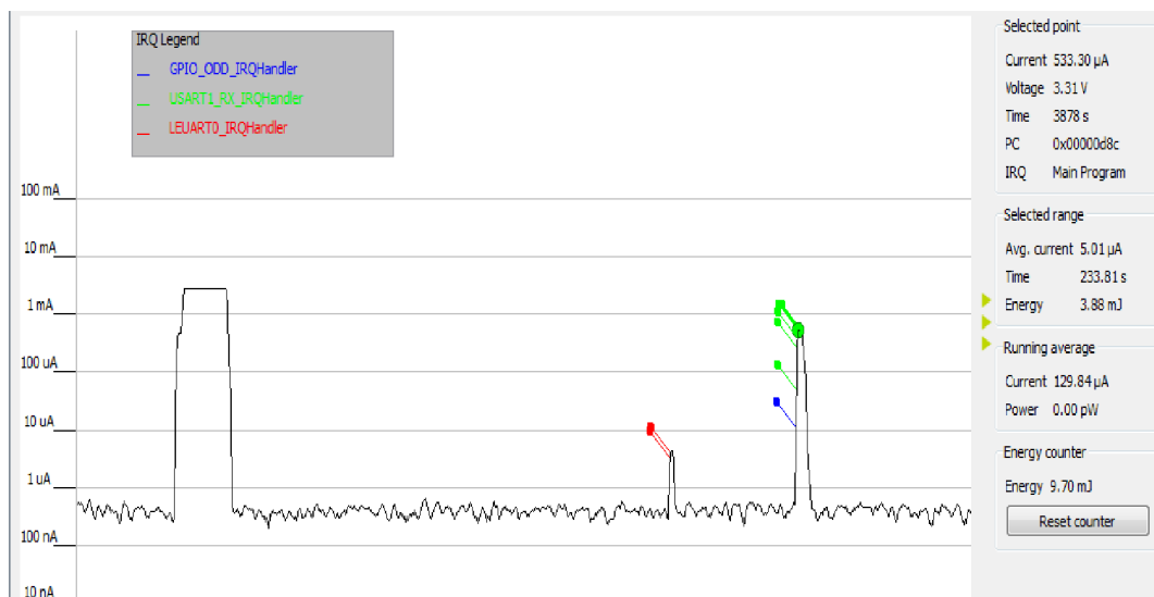
Obr. 4-19 Meranie spotreby prúdu LEUART a UART
