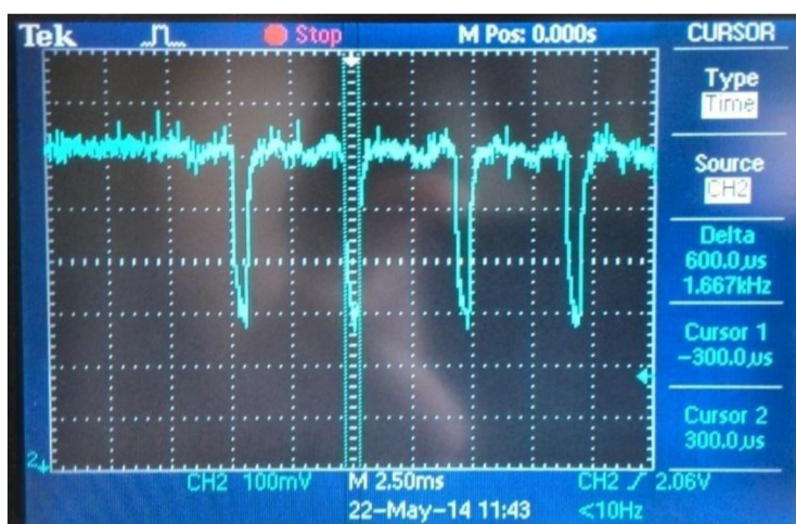
Obr. 4-24 Dĺžka trvania burst rámcov
