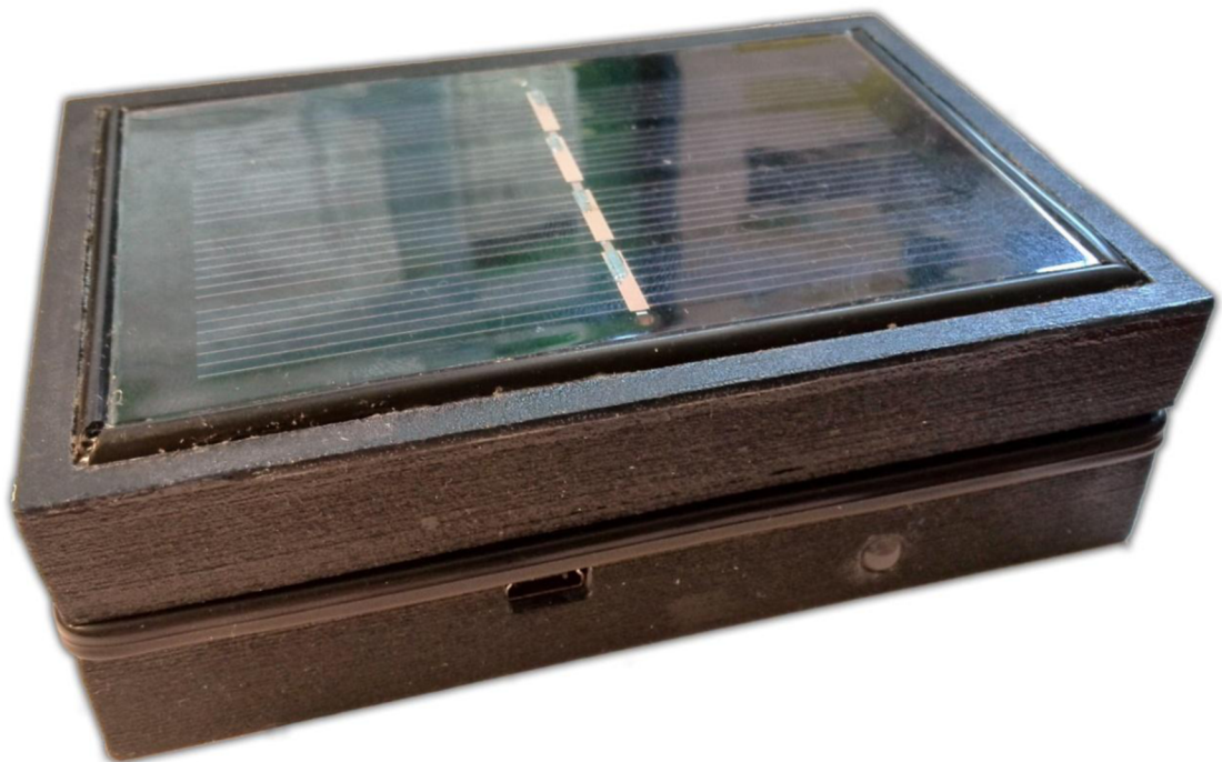
Obr. 5-23 Hotový nízkoenergetický senzorový modul - zatvorený
