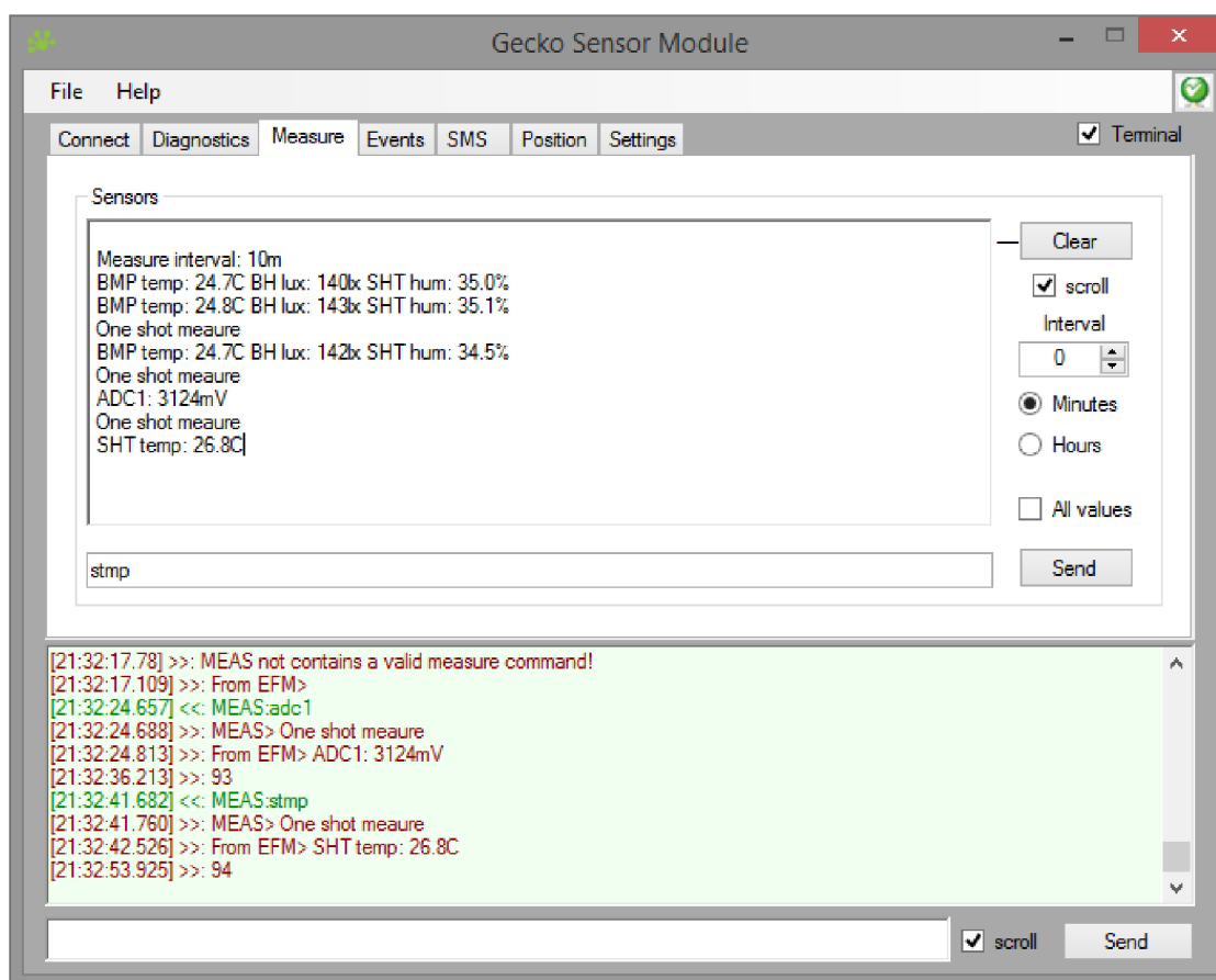
Obr. 4-10. GUI - okno pre lokálne meranie
