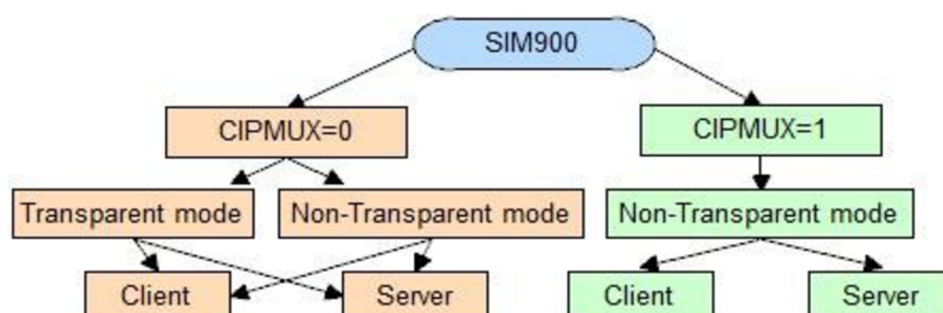
Obr. 3-7 SIM900 štruktúra TCP/IP podľa [22]
