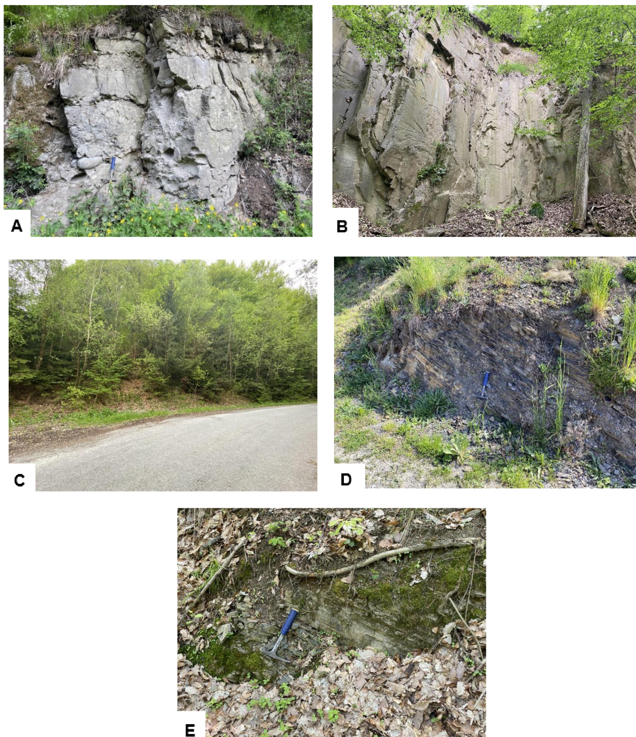
Obr. 14: Paleontologické lokality myslejovického souvrství s výskytem gastropodové fauny. A – Opatovice 6, výchozy se střídajícími se polohami slepenců a drob; B – opuštěný drobový lom na lokalitě Opatovice 6; C – Opatovice 12, odkryv břidlic a drob podél cesty k domku hrázného; D – Pístovice Š, výchoz podél cesty ke staré škole; E – Pístovice Ž, skalka podél potůčku, vlévajícího se do Pístovického rybníka.
