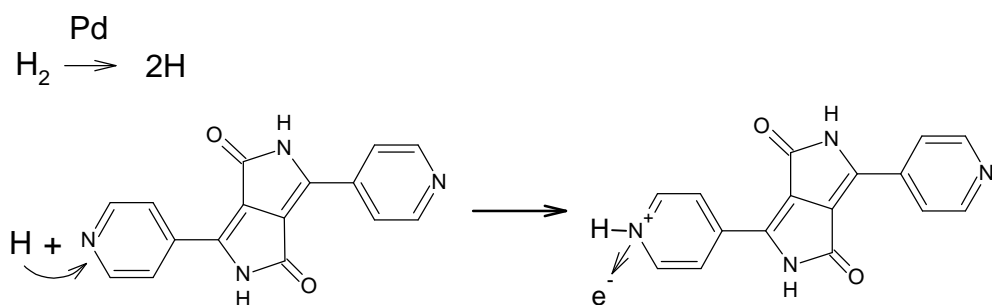
Obr. 2 Reakční schéma
