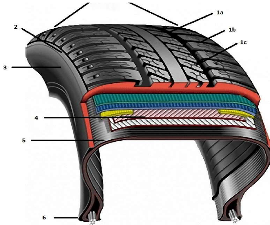
Obrázek 1 Konstrukce pneumatiky
