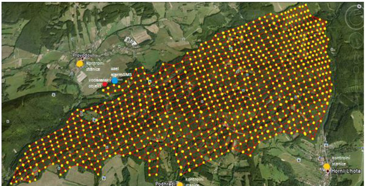
OBRÁZEK 17 - TOPOLOGIE SÍŤE
