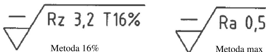
Obr. 12) Označování drsnosti povrchu na výkrese podle ISO 1302 [17]
