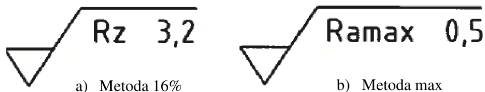
Obr. 12) Označování drsnosti povrchu na výkrese podle ISO 1302 [17]
