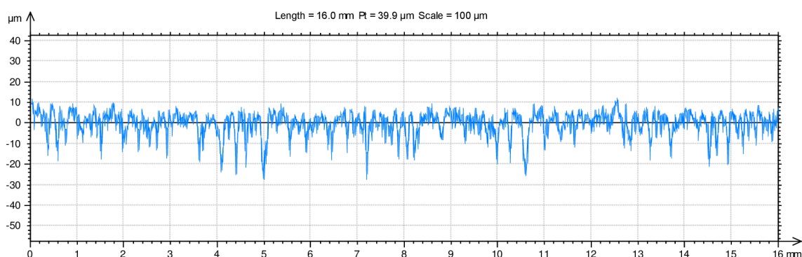
Obr. 22) Zavedení filtru \lambda f
