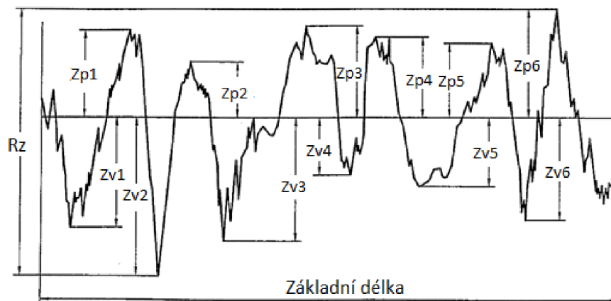
Obr. 9) Největší výška profilu drsnosti [15]
