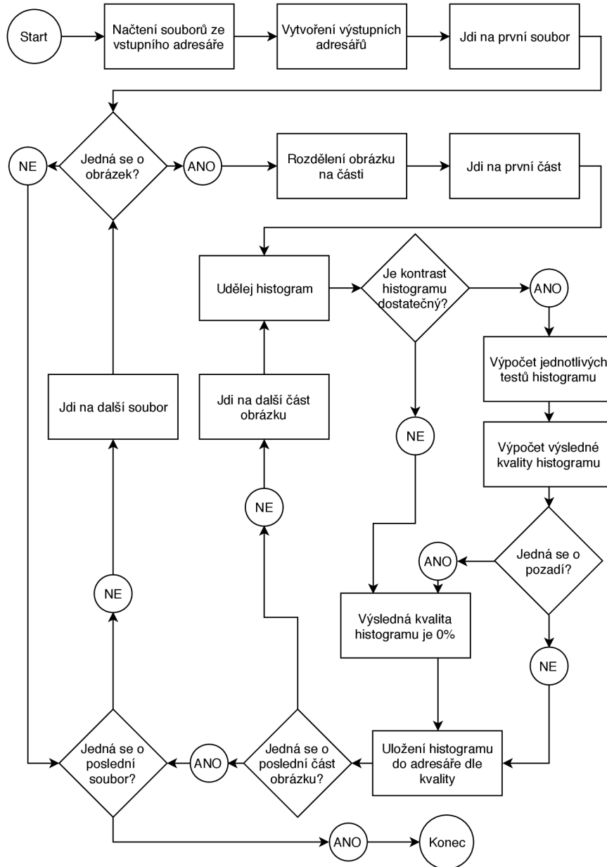
Obrázek 4.1: Vývojový diagram – návrh fungování celého skriptu
