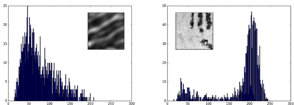
Obrázek 3.3: Tmavý obrázek a histogram, světlý obrázek a histogram.
