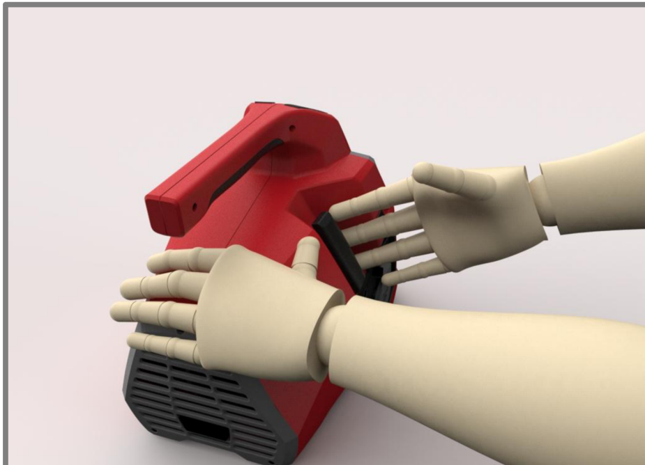
Obr. 6-24 Startování generátoru
