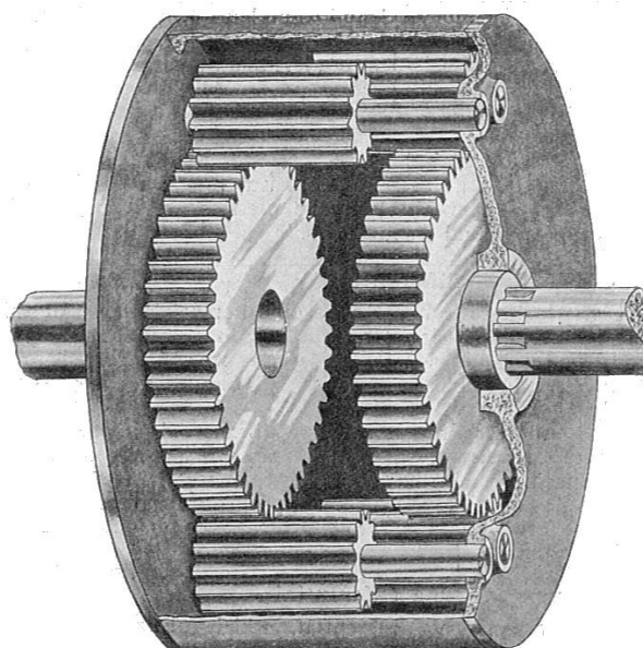
Obrázok 4 Čelný diferenciál [5]
