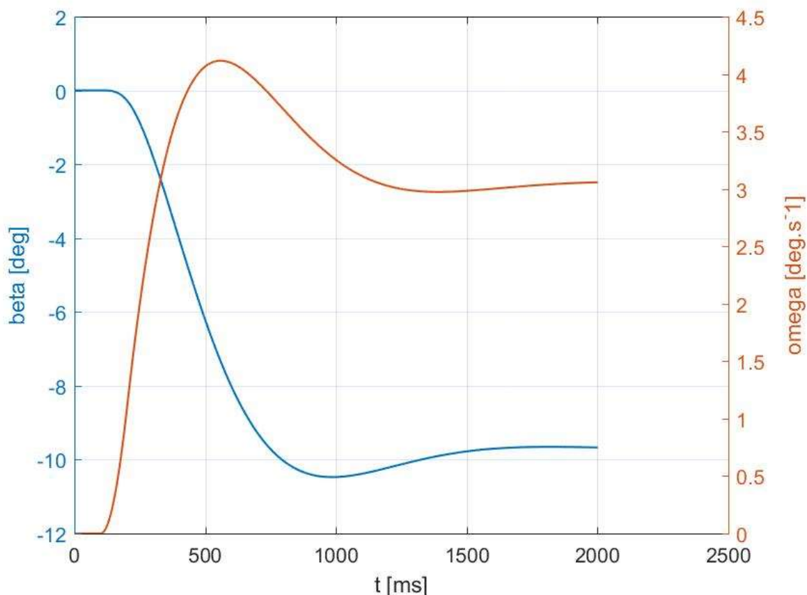
Obrázok 18 Závislosť uhlu smerovej odchýlky a stáčiavej rýchlosti na čase
