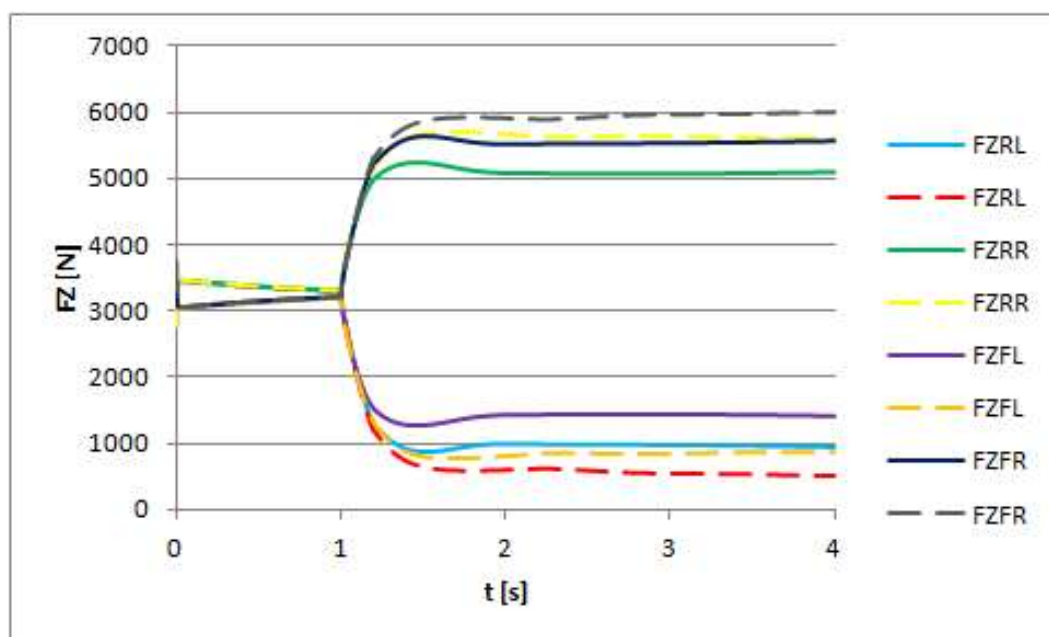
Obrázok 32 Zvislá sila v závislosti na čase – natočenie 6°
