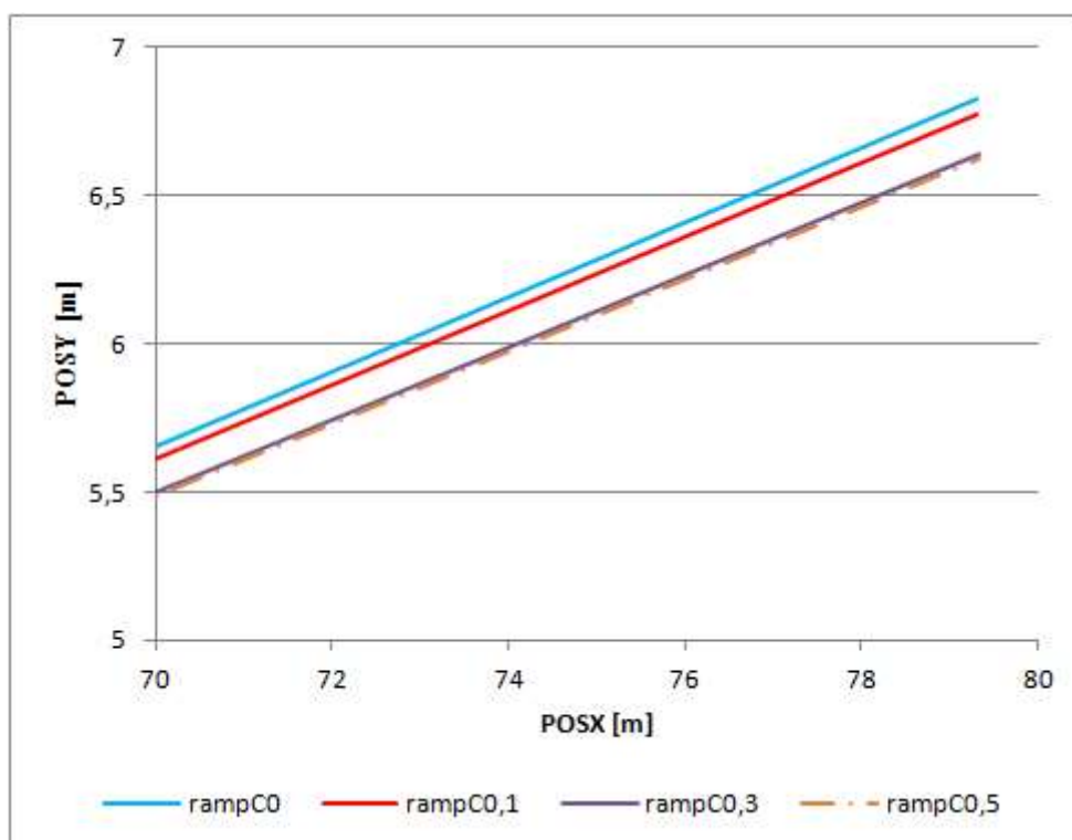
Obrázok 50 Trajektória vozidla – priblíženie, nulové predpätie
