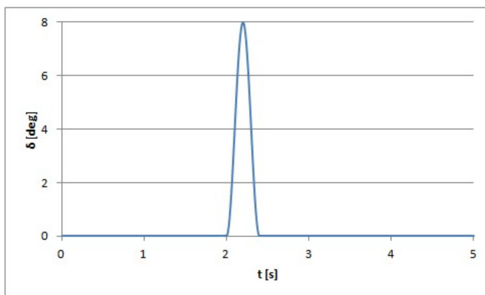
Obrázok 44 Priebek natočenia volantu – maximum 8^\circ
