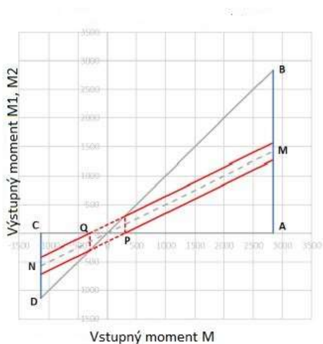
Obrázok 39 Výstupné momenty v závislosti na privedenom momente – predpätie [11]
