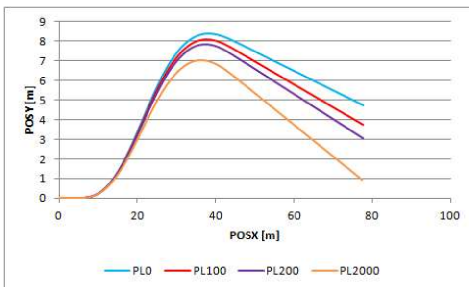
Obrázok 59 Trajektória vozidla
