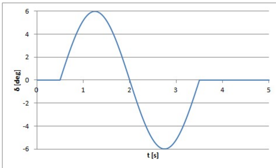
Obrázok 53 Priebeh natočenia volantu – maximum 6^\circ
