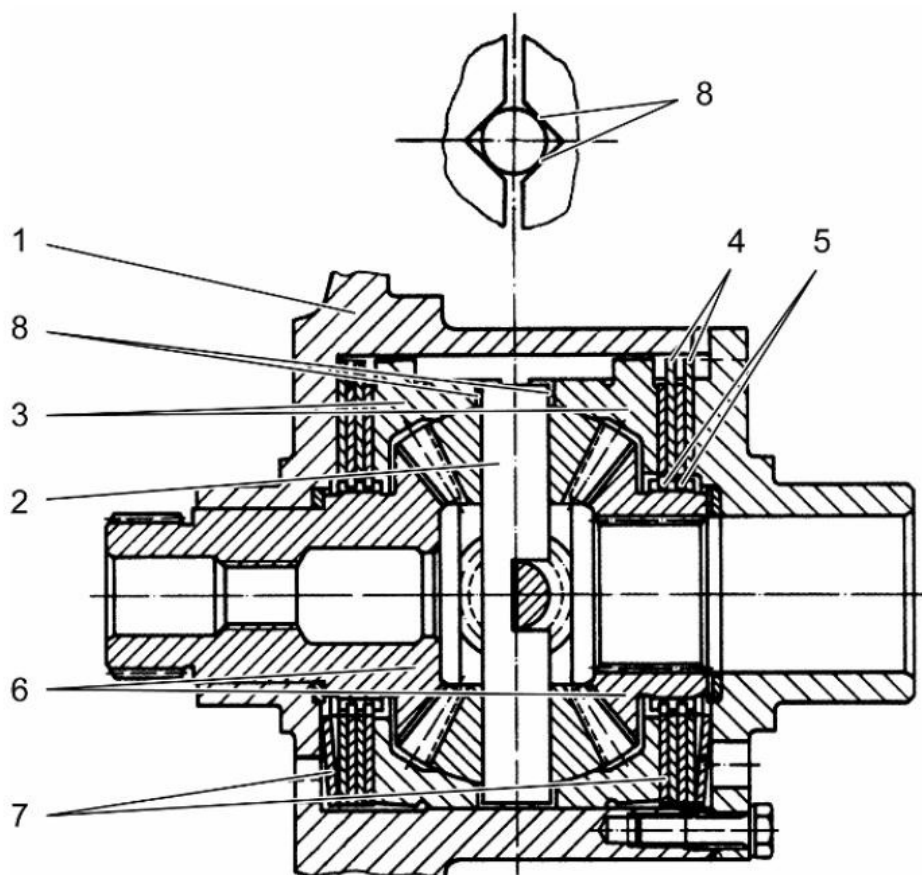
Obrázok 7 Diferenciál Lok-o-matic – horná časť bez predpätia , dole s predpäťm [7]
