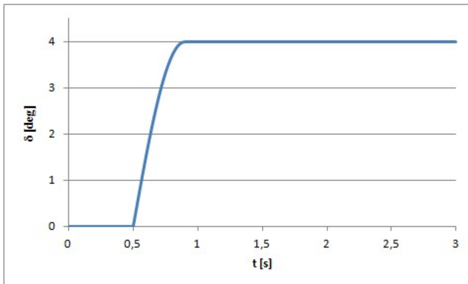
Obrázok 60 Natočenie predných kolies počas menévru
