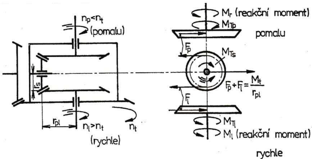
Obrázok 5 Kinematické a silové pomery na diferenciálu so zvýšeným trením[3]
