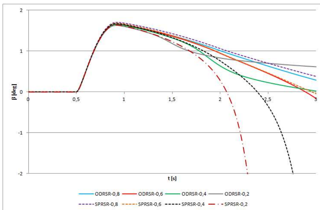
Obrázok 64 Uhol smerovej odchýlky – zadný pohon
