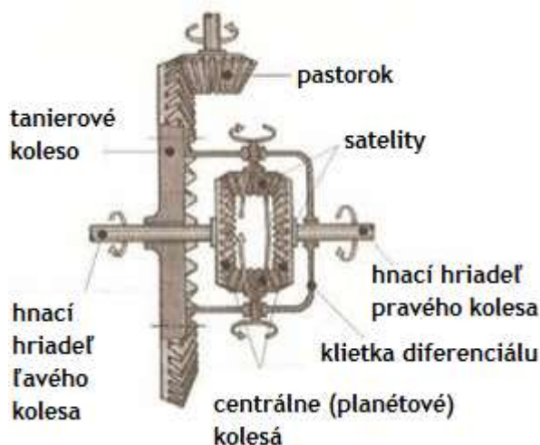
Obrázok 1 Kužel'ový diferenciál [2]
