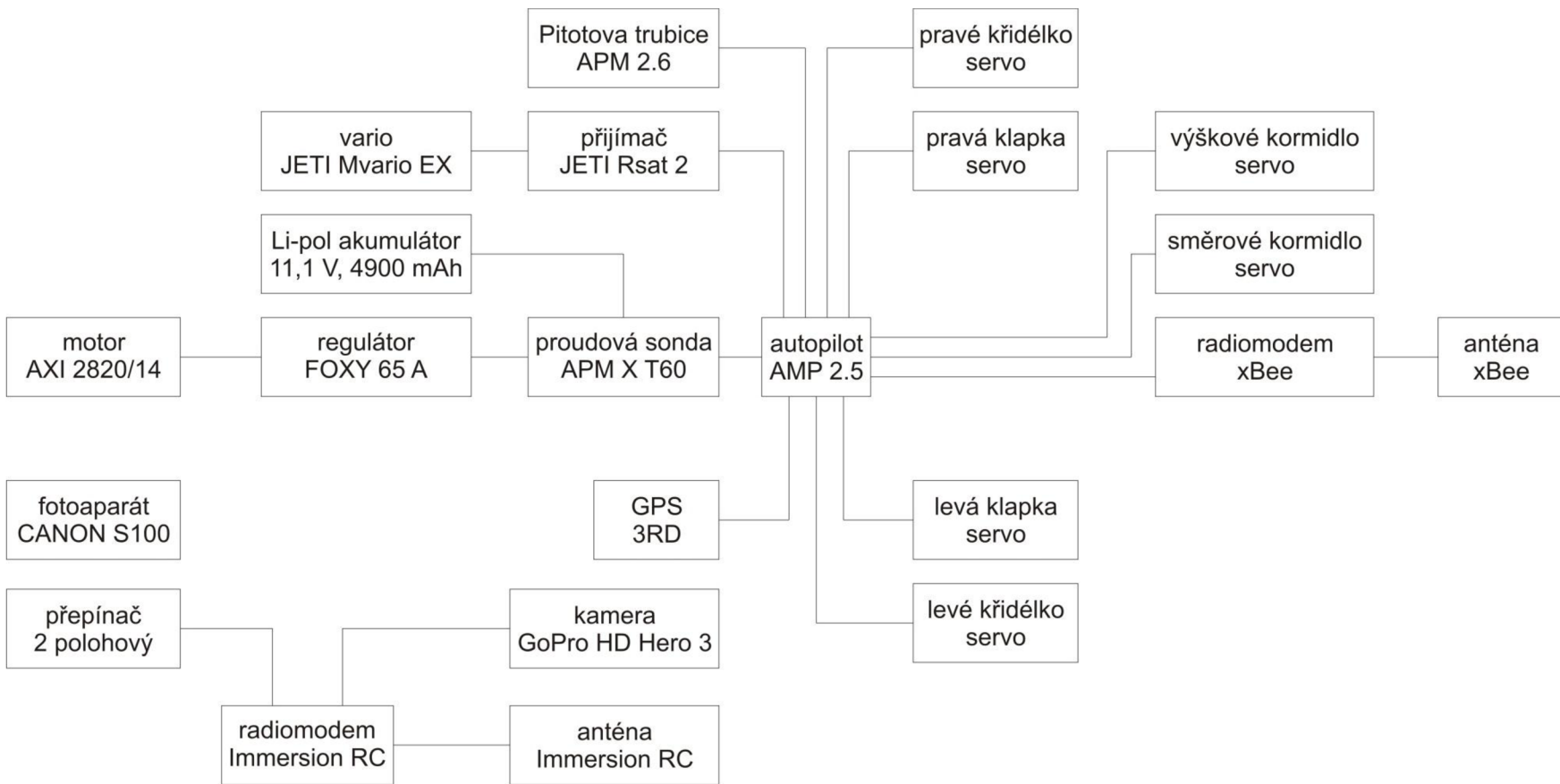
Příloha 2: Blokové schéma zapojení palubní elektroniky letounu Multiplex Cularis
