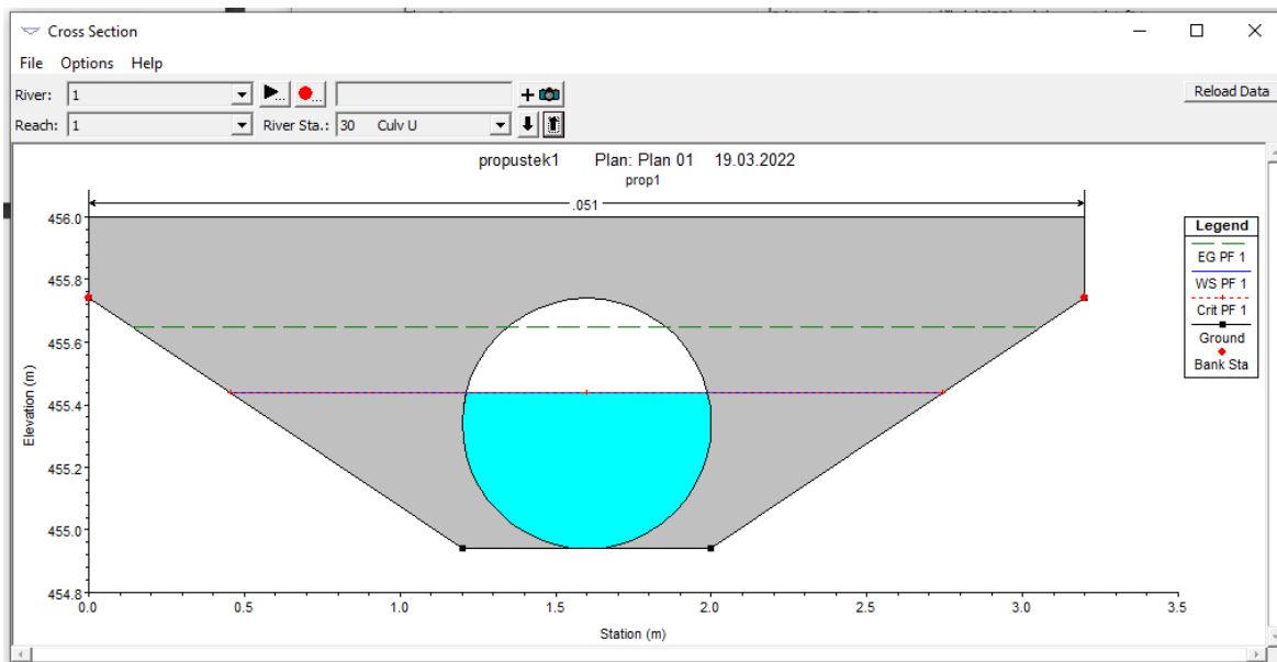
Obrázek 5-14 Příklad příčný řez ve staničení km 0,02999, hloubka 0.5 m. Program hec ras.
