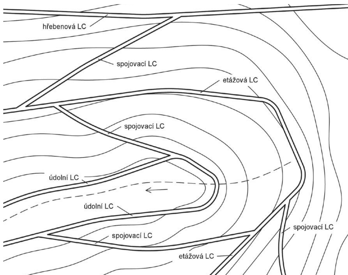
Obrázek 3-1 Struktura lesních cest v údolí. Zdroj: TD LDS
