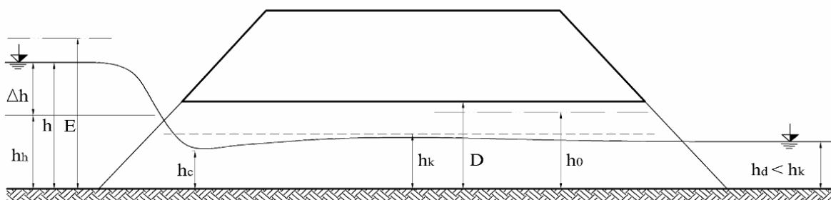
Obrázek 3-11 Schéma propustku o volné hladině neovlivněného spodní vodou.
