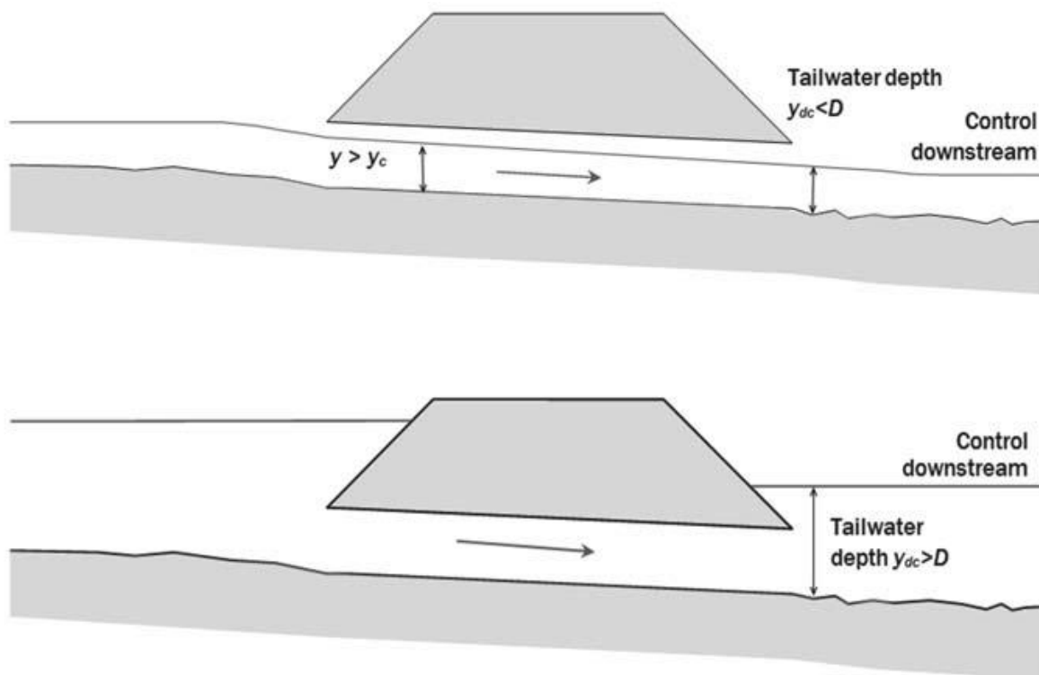
Obrázek 3-6 Příklad propustku s kontrolou výtokem. Zdroj: Hydraulic Design of Highway culverts 2012. Fig 6.8
