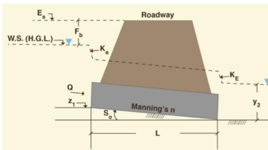
Obrázek 4-13 Schematický obrázek vstupních parametrů. Kalkulátor online culvert
