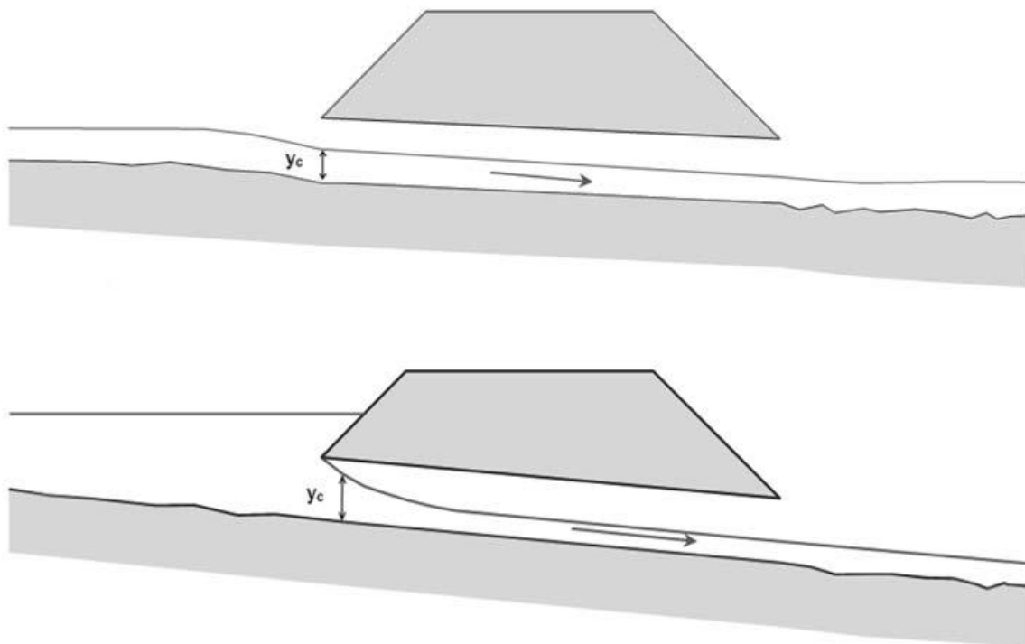
Obrázek 3-5 Příklad propustku s kontrolou vtokem. Zdroj: Hydraulic Design of Highway culverts 2012. Fig 6.7
