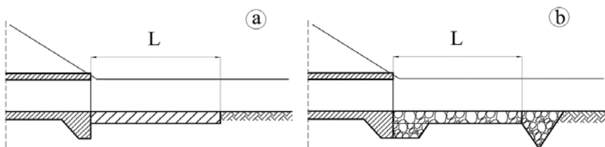
Obrázek 2-23 Spadiště za propustkem. Zdroj: TP 204
