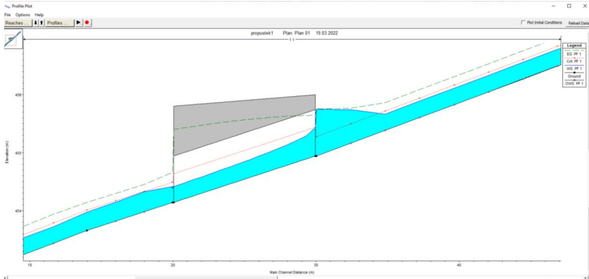
Obrázek 5-10 Podélný profil proudění v trase. Program HEC-RAS.
