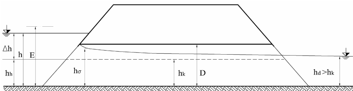
Obrázek 3-15 Schéma propustku se zahlceným vtokem ovlivněného dolní vodou.
