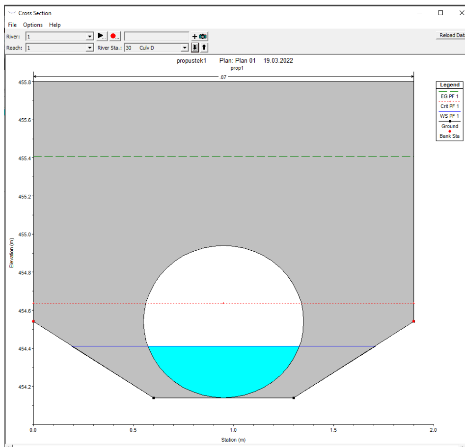
Obrázek 5-15 Příklad příčný řez ve staničení km 0,02001, hloubka 0.27 m. Program hec ras.
