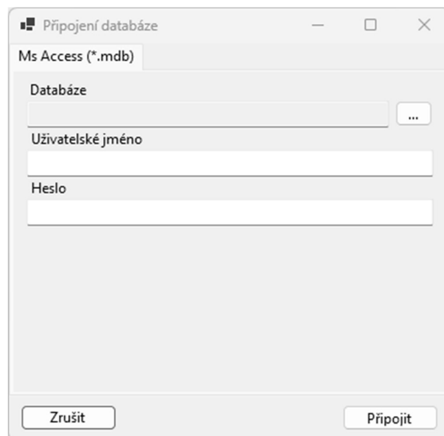
Obrázek 9 - Okno připojení
