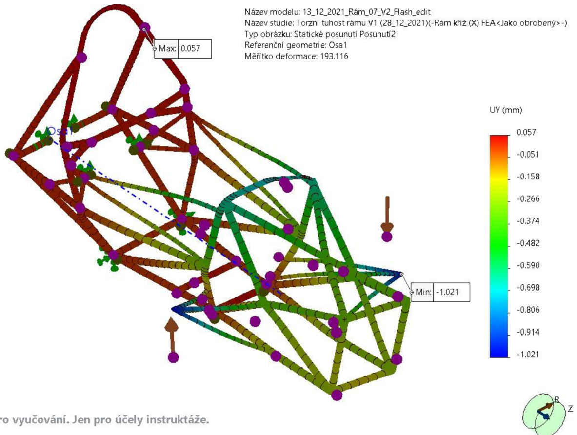
Obrázek 2 Výsledky pevnostní simulace rámu – Varianta č.2 [Archiv autora]
