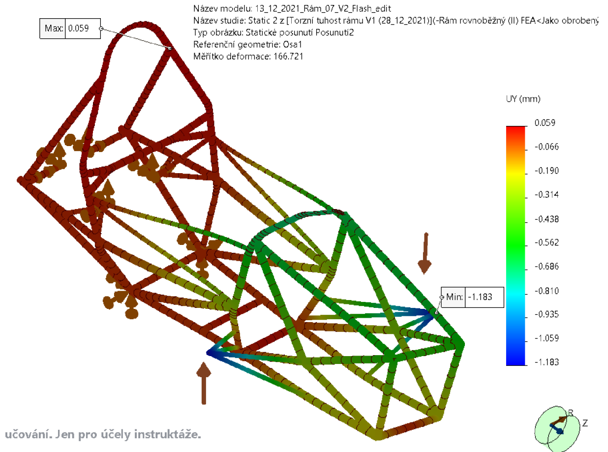
Obrázek 1 Výsledky pevnostní simulace rámu – Varianta č.1 [Archiv autora]
