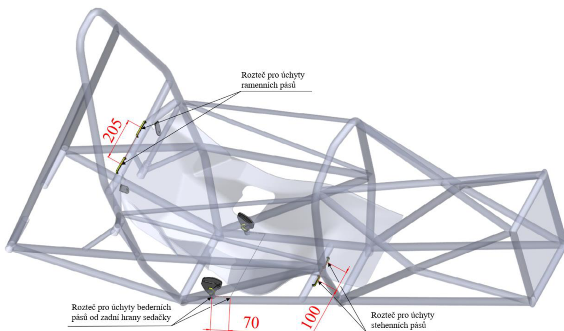
Obrázek 21 Pozice úchyťů pásů na monopostu FS07 [Archiv autora]
