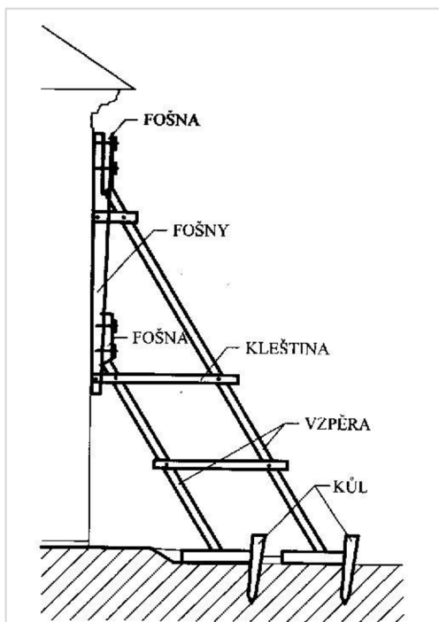
Obrázek 4: Provizorní podchyčení zdiva
