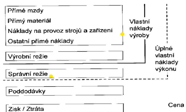
Obrázek 8: Kalkulační vzorec
