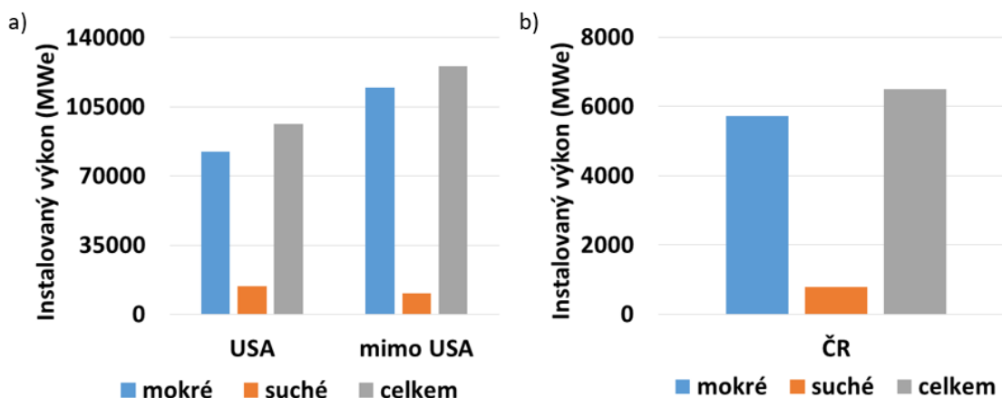
Obr. 2.4: Rozšíření odsiřovacích technologií podle instalovaného výkonu uhelných elektráren: a) údaje k roku 1998 z [20], b) údaje pro ČR k roku 2006 z [5]).
