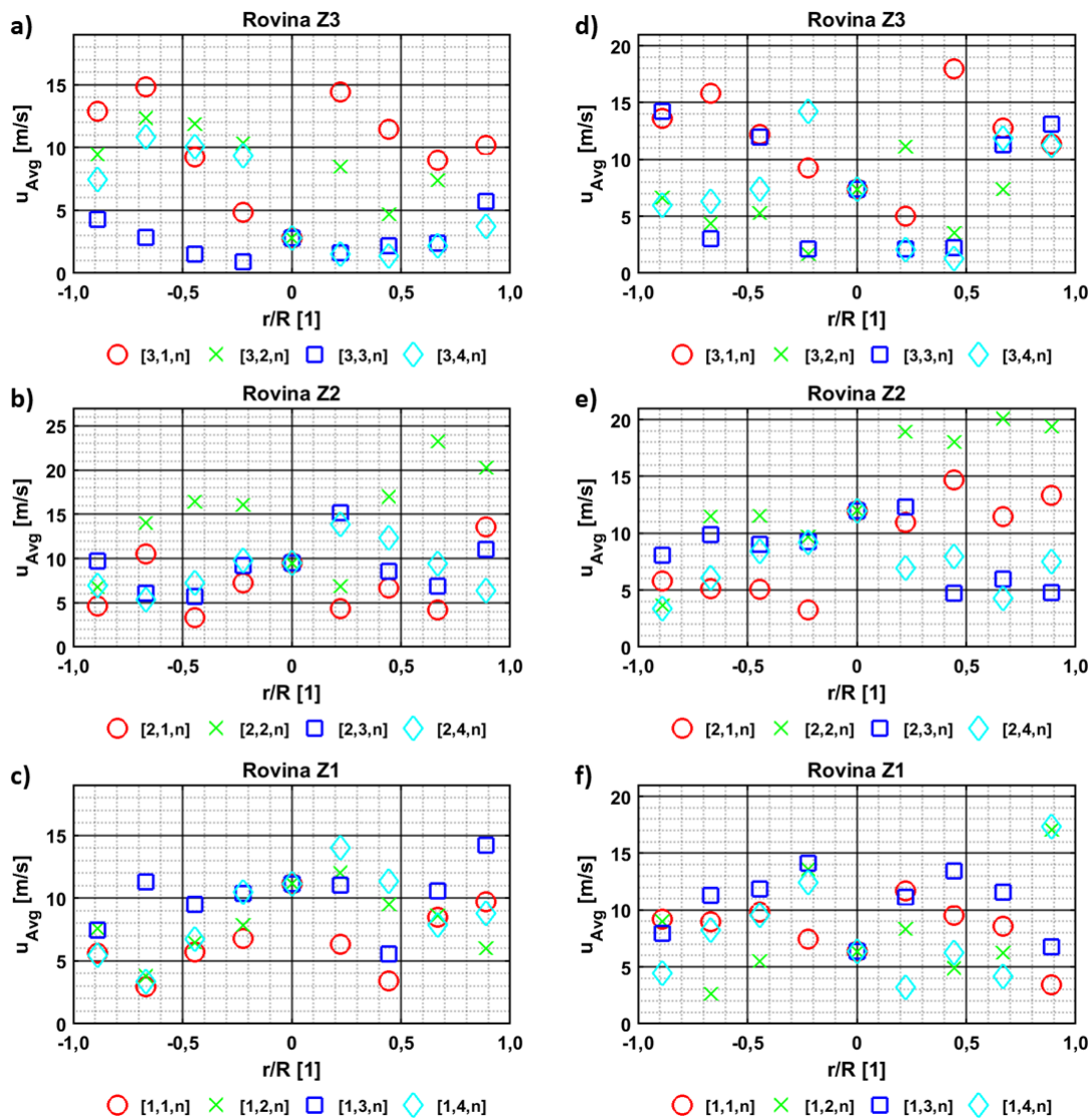
Obr. 5.8: Rychlostní profily – režim III: a, b, c) 40% výkon ventilátoru, d, e, f) 70% výkon ventilátoru.
