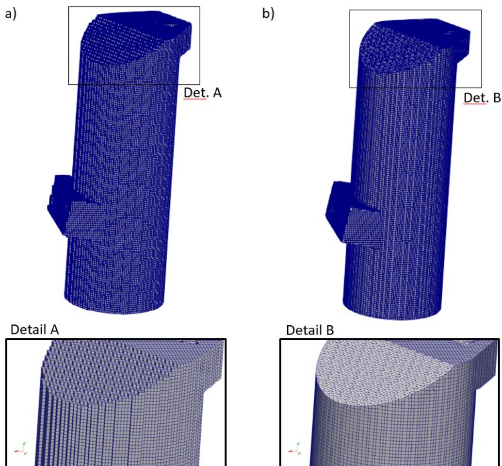
Obr. 6.5: Postup tvorby sítě pomocí snappyHexMesh : a) krok 1, b) krok 2.
