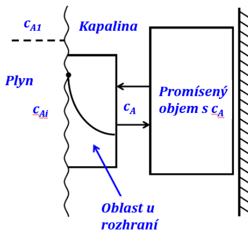
Obr. 3.5: Přenos hmoty s chemickou reakcí – ilustrace profilů koncentrace (převzato z [34]).
