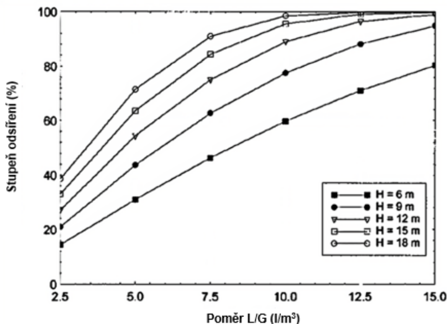
Obr. 4.1: Účinnost odsíření v závislosti na poměru L/G a výšce absorpční zóny (převzato z [43]).
