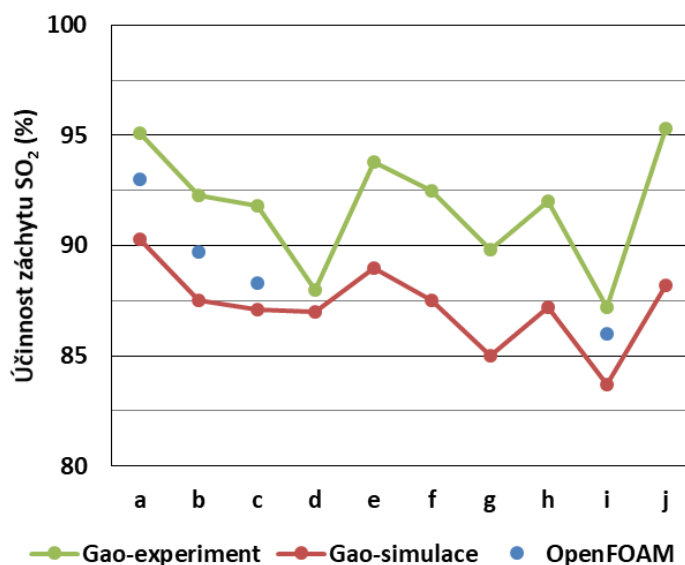
Obr. 6.23: Reaktor pro jednoduchou úlohu – porovnání účinnosti zachytu SO 2 s prací Gaa [44].
