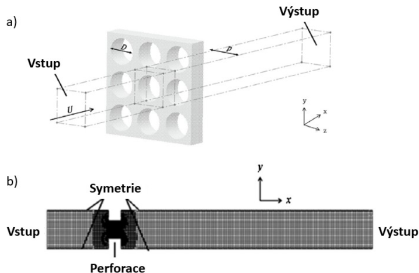
Obr. 4.7: Jednotková buňka perforovaného plechu: a) náčrtek, b) výpočetní síť s OP (převzato z [60]).
