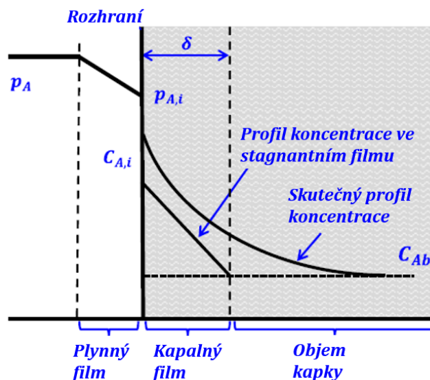
Obr. 3.2: Filmová teorie – schématické znázornění filmů v blízkosti rozhraní (převzato z [34]).
