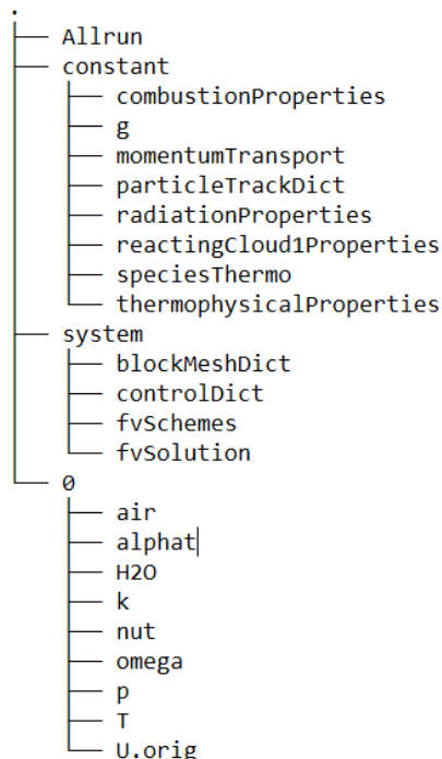
Obr. 6.2: Úloha verticalChannel – adresářová struktura.
