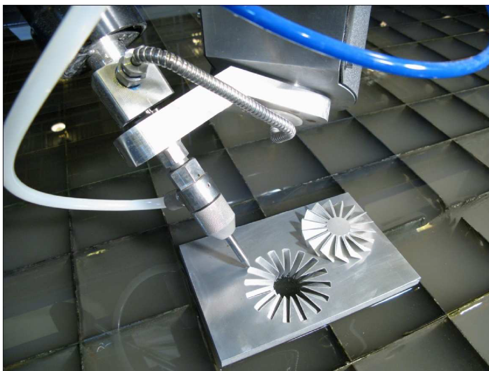
Obr. 2.26 Řezání pomocí 5-osé řezací hlavy firmy WARDJet Psy
