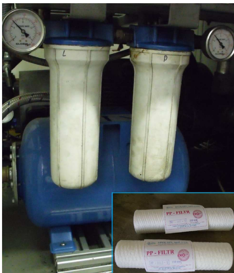
Obr. 5.2 Vodní filtry - umožňují recyklaci vody
