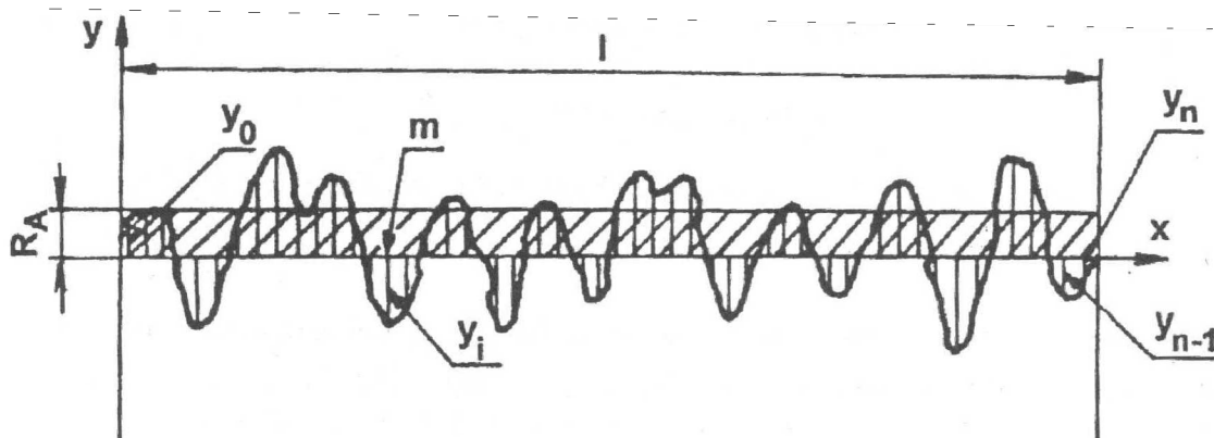
Obr. 4.12 Střední aritmetická odchylka profilu - R_a [43]
