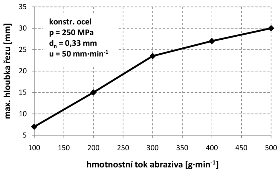
Obr. 4.5 Vliv hmotnostního abrazivního toku na hloubku řezu [4]
