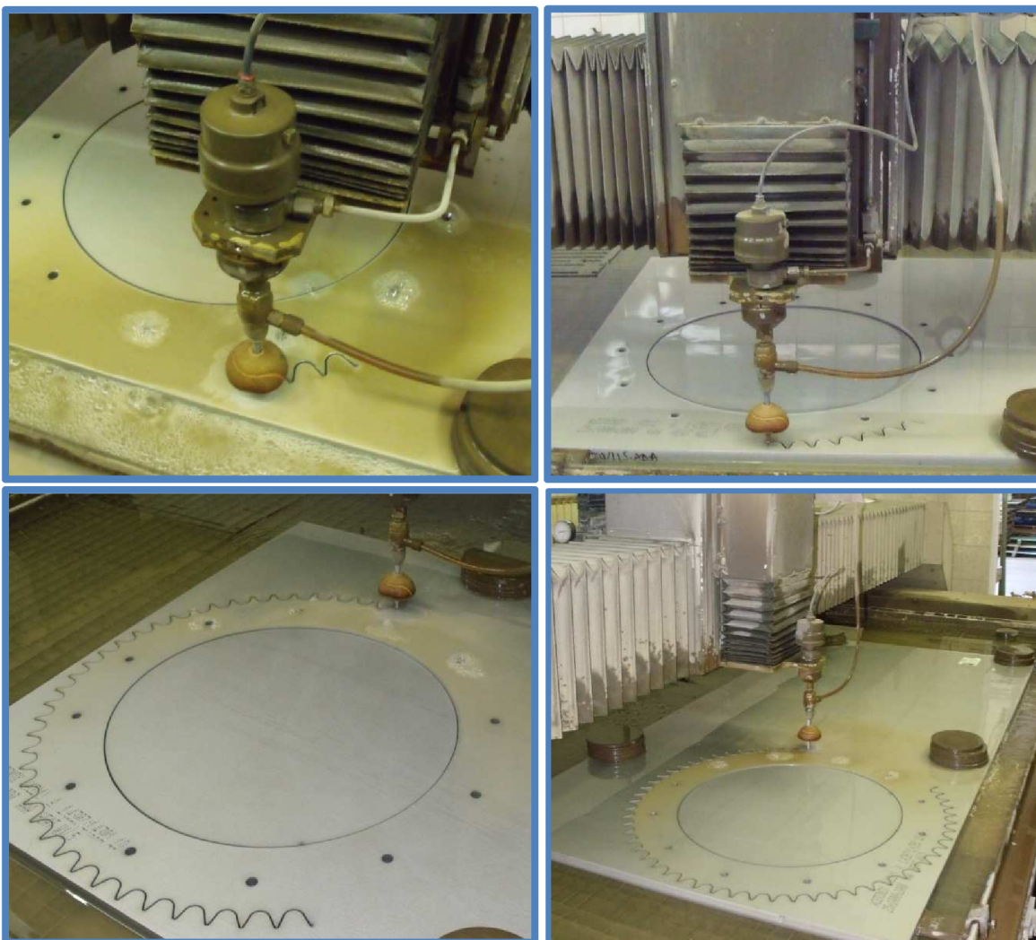
Obr. 6.15 Řezání zubů řetězového kola (výkres F 74 13332; 61 zubů)
