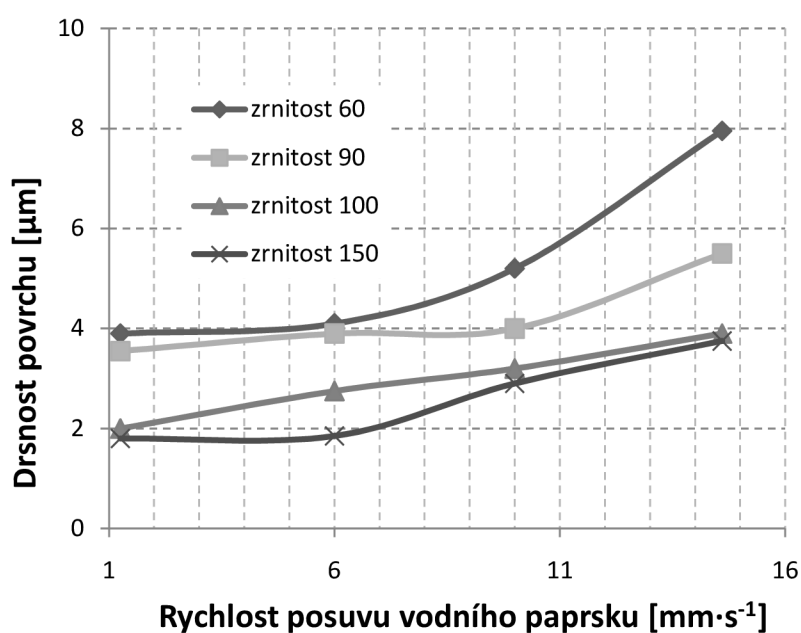
Obr. 4.14 Vliv velikosti částic brusiva na drsnosti povrchu. Podmínky řezání: m_a=7,6 g·s -1 ; průměr dýzy 0,330mm; tlak = 311MPa; granát; obrobek: Inconel 718 [7]
