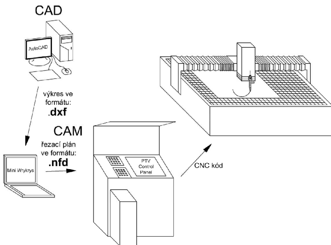
Obr. 3.1 Zadávání a řízení výroby pomocí CAD/CAM technologií
