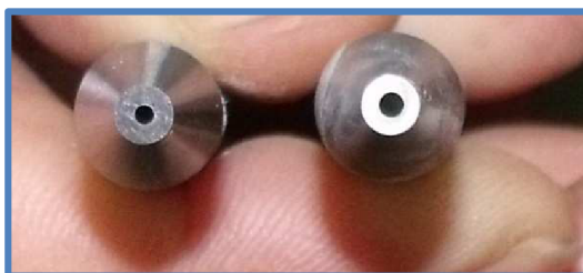
Obr. 6.9 Nová zaostřovací trubice (vlevo), stará zaostřovací trubice
