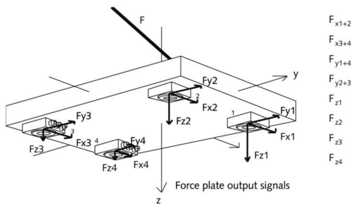
Obr. 25 Znáornění sil desky tvořící výstupní signál (Kistler Group, 2008)
