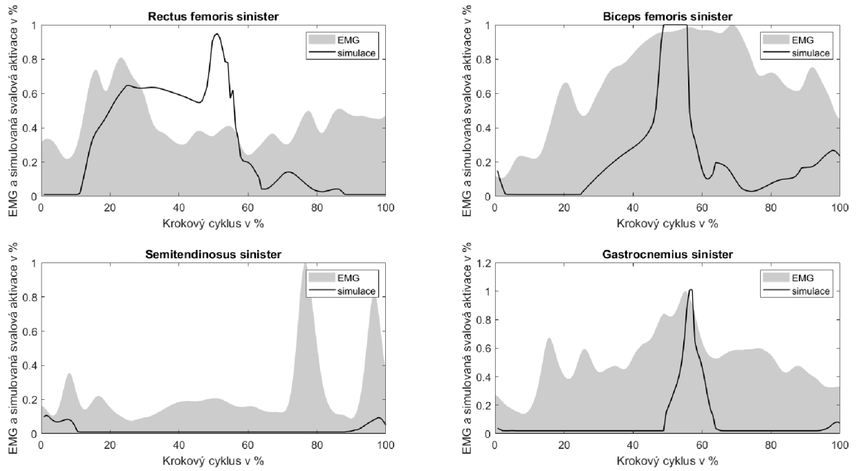
Graf 31 Porovnání EMG a simulované svalové aktivace pro levou končetinu při chůzi respondenta A bez ortézy (Zdroj: autor)
