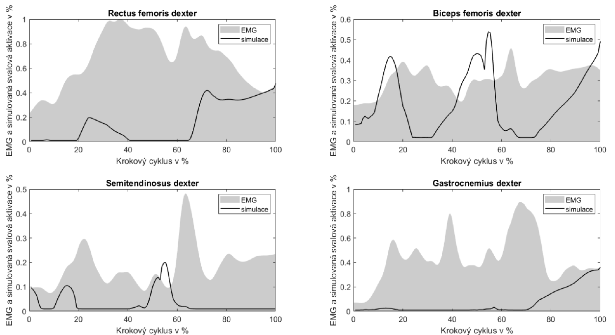
Graf 32 Porovnání EMG a simulované svalové aktivace pro pravou končetinu při chůzi respondenta A bez ortézy (Zdroj: autor)
