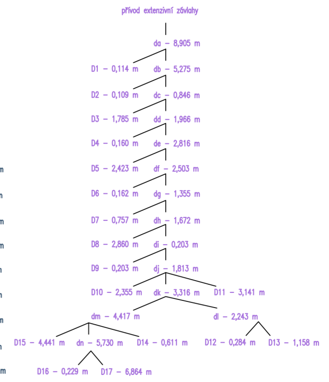
FUNKČNÍ SCHEMA ZAPOJENÍ EXTENZIVNÍ ZÁVLAHY
