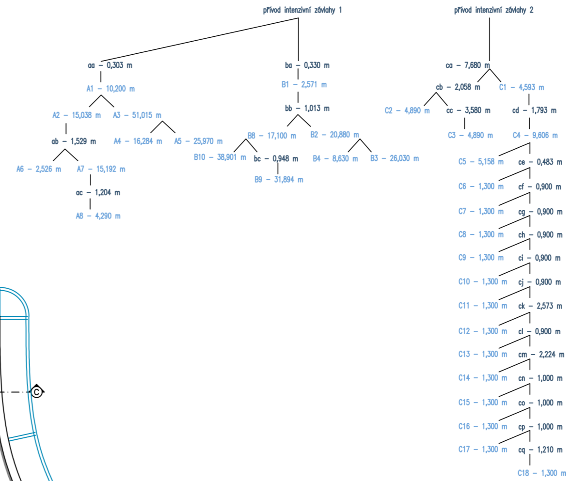
FUNKČNÍ SCHEMA ZAPOJENÍ INTENZIVNÍ ZÁVLAHY
