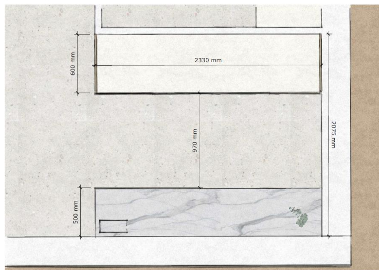
Púdorys kuchyne c.2
