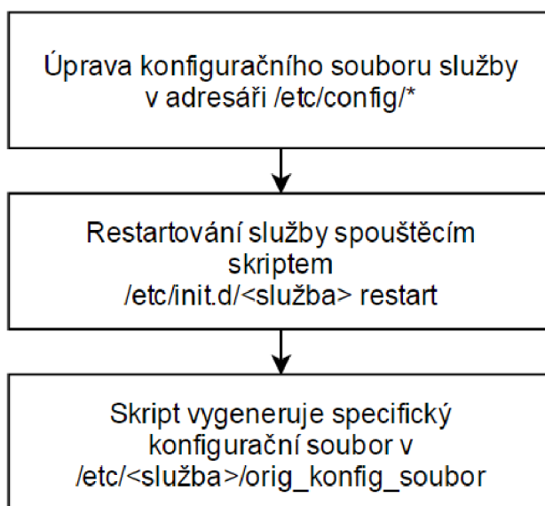
Obr. 3.1: Modifikované konfigurační soubory UCI se při restartu služby převedou do konfiguračního souboru specifické služby.
