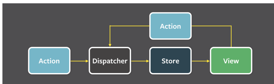
Obrázek 3: Flux: Data flow diagram [25]
