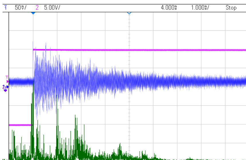
Obr. 7-9: Zmeraný signál z piezoaktuátora pri identickej zostave.
