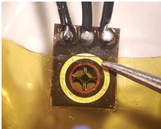
Obr. 7-4: Izolácia otvoru membrány kaptonovou páskou (TDK ICS-40730)
