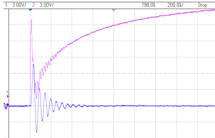
Obr. 6-4: Zákmyty a oscilácie počas nábehu napätia.
