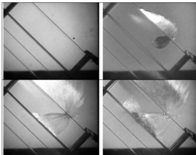
Obr. 2-1: Efekt HVI na Whippleov štít [6]
