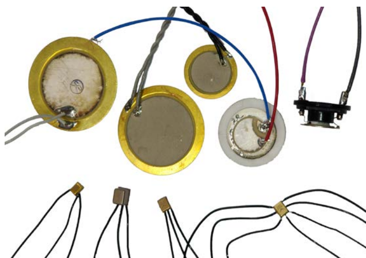
Obr. 7-2: Snímok väčšiny použitých snímačov s výnimou piezofólií
