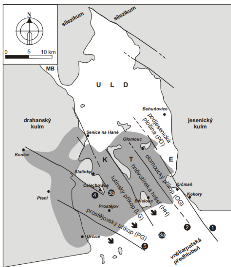
Obr. 3 Strukturně-geologické schéma území severní části Hornomoravského úvalu (HMU); zdroj: Jan Zapletal; dostupné z: https://journals.muni.cz/gvms/article/view/4904
