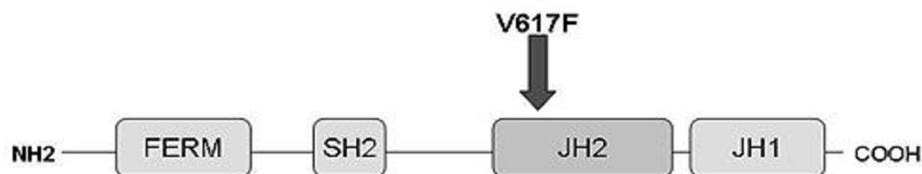
Obrázek 1: Schéma mutace JAK2 V617F .
