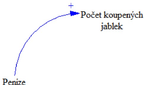
Obrázek 4: Kladná vazba
