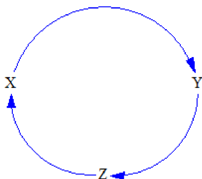
Obrázek 2: Systemové myšlení
