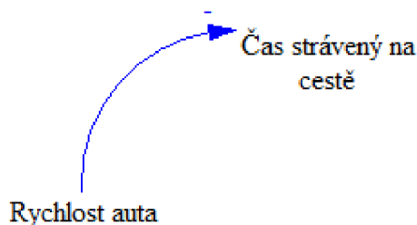
Obrázek 5: Záporná vazba
