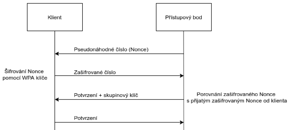
Obrázek 2.2: Autentizace WPA-Personal [17]
