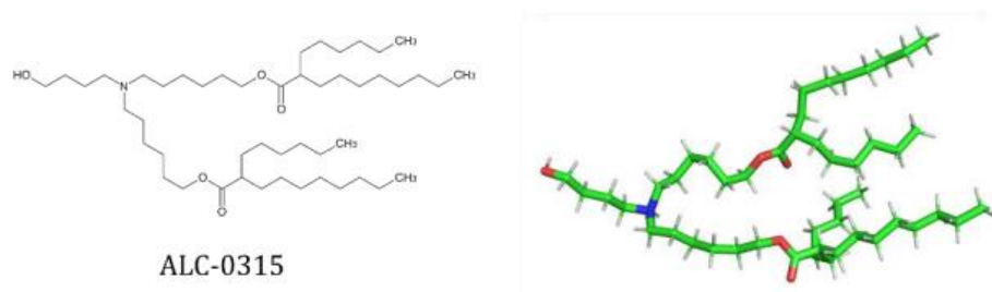
Obrázek 3: chemická struktura a 3D vizualizace ionizovatelného lipidu ALC-0315 (c)
