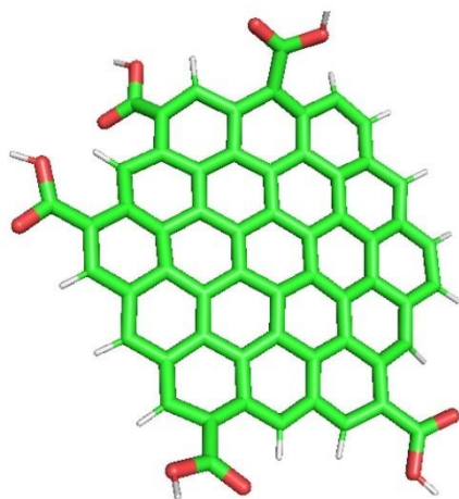
Obrázek 7: C3-karboxyl
