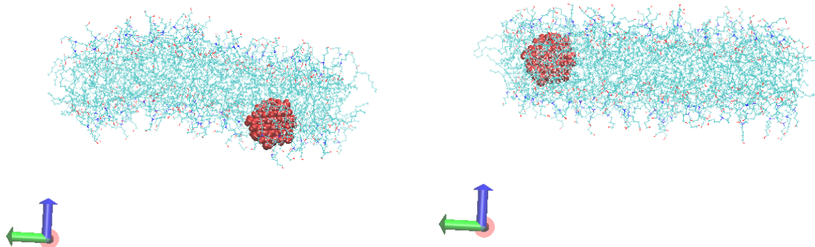
Obrázek 9: série snímků dynamického pohybu modelu vrstvy uhlíkové tečky C3-amin
