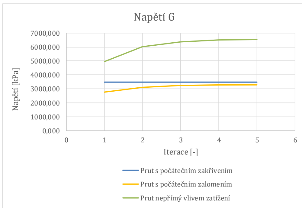
Obr. 4. 10 Grafické znázornění iterací napětí pro jednotlivé typy prutů – 40% F_{cr}
