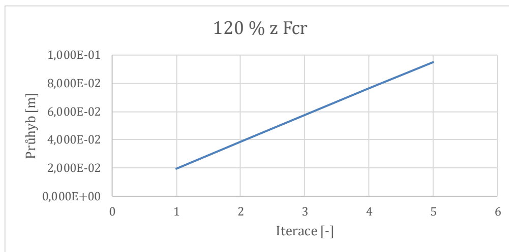
Obr. 4. 19 Grafické znázornění iterací průhybů – 120% Fcr
