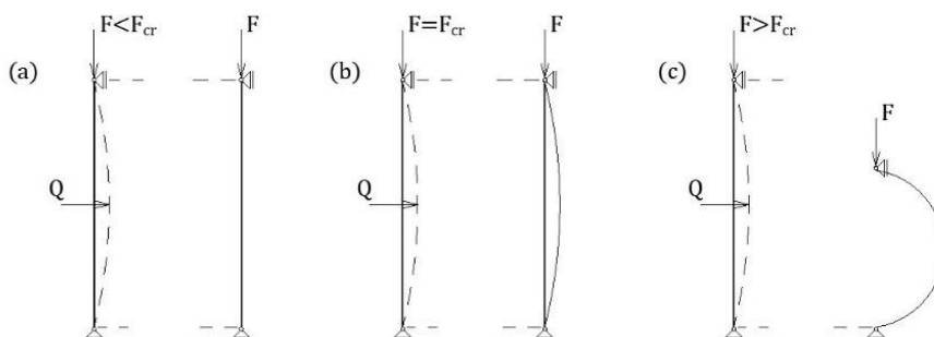
Obr. 2. 1 Stabilní, indiferentní a nestabilní stav tlačенého ideálního prutu
