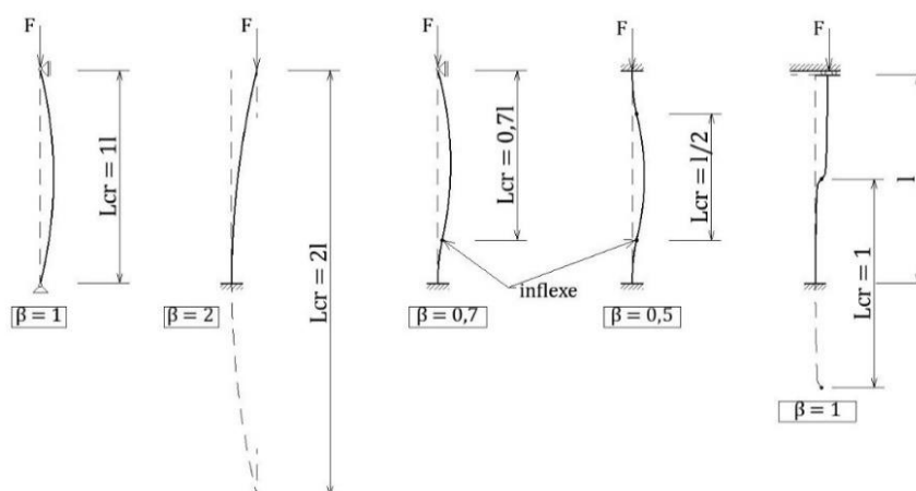
Obr. 2. 2 Přehled základních Eulerových případů, vzpěrné délky [1]
