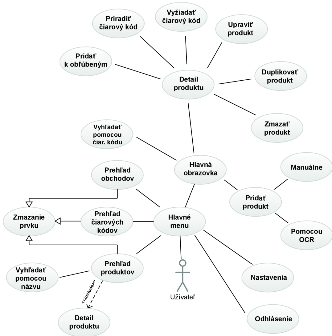
Obrázok 2.1: Diagram prípadov použitia pre aplikáciu
