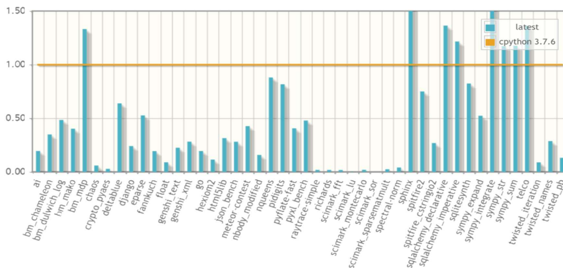
Obr. 4: Porovnání časů testů pro PyPy a CPython [13]
