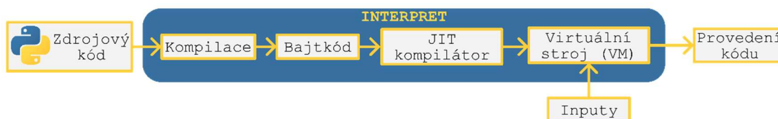
Obr. 2: JIT interpret
