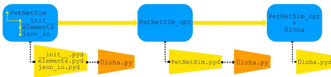
Obr. 19: Proces úpravy úloh před kompilací
