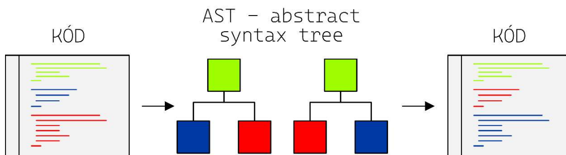
Obr. 8: Schéma transpileru [24]
