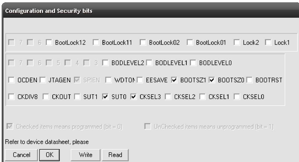
Obr. 16: nastavení bezpečnostních a konfiguračních zámků v programu Pony Prog
