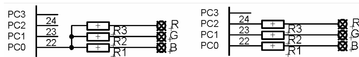
Obr. 4: Zapojení pro monochromatický a barevný obraz
