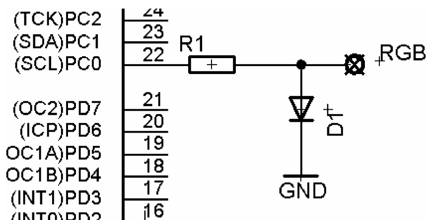
Obr. 2: Napojení barevného signálu na výstupní port
