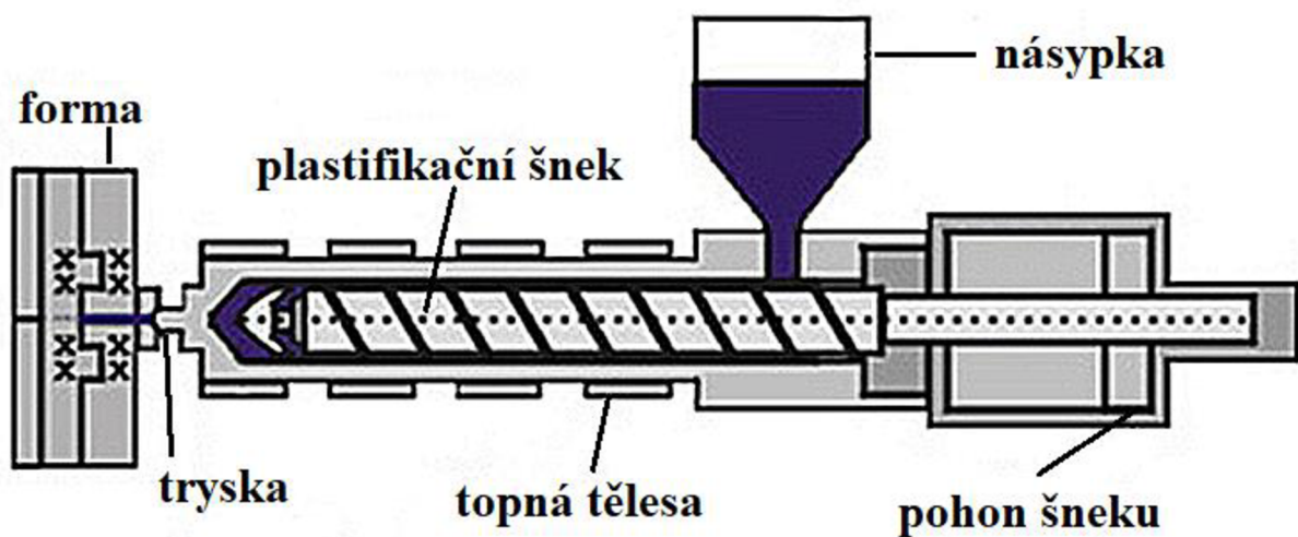
Obr. 13 Vstřikovací jednotka [18]
