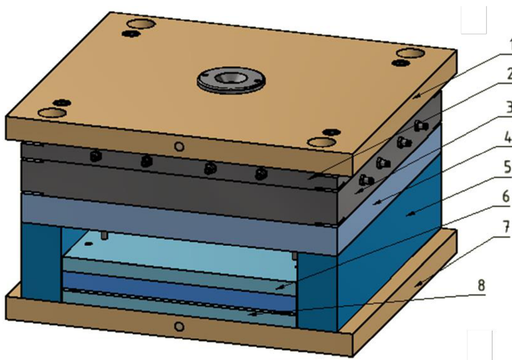
Obr. 43 Základní díly vstřikovací formy [22]
