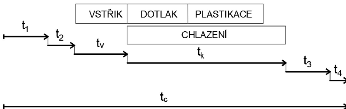
Obr. 36 Znáornění vstřikovacího cyklu [25]
