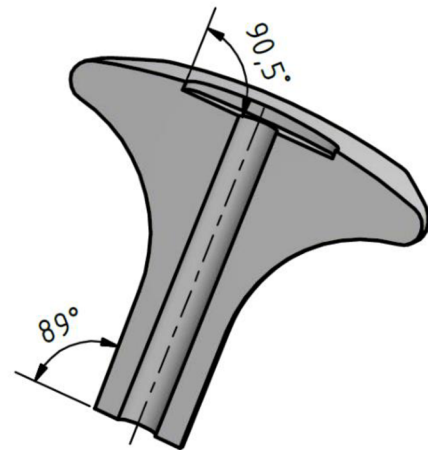
Obr. 34 Technologické úkosity
