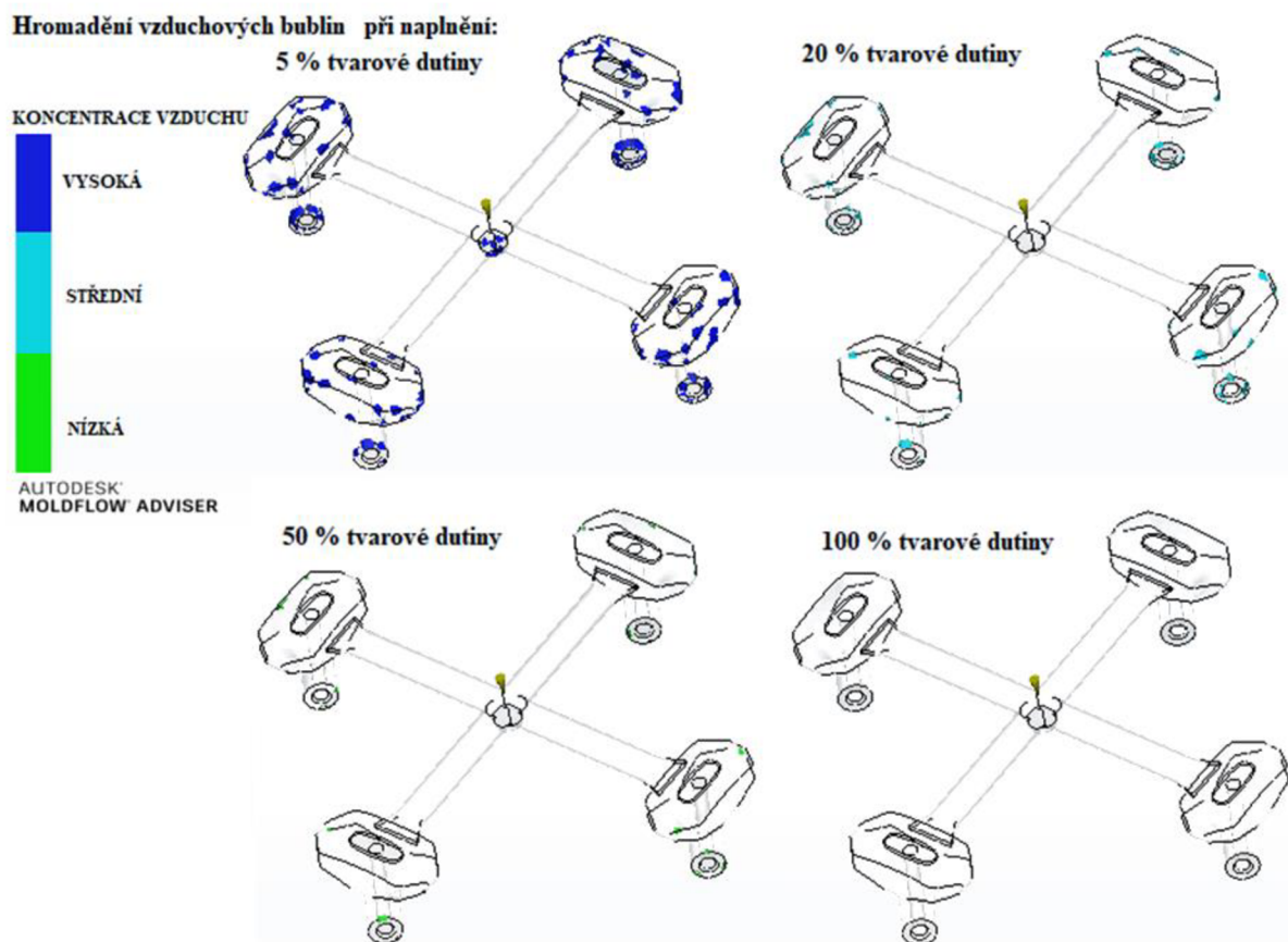
Obr. 42 Hromadění vzduchu ve tvarové dutině
