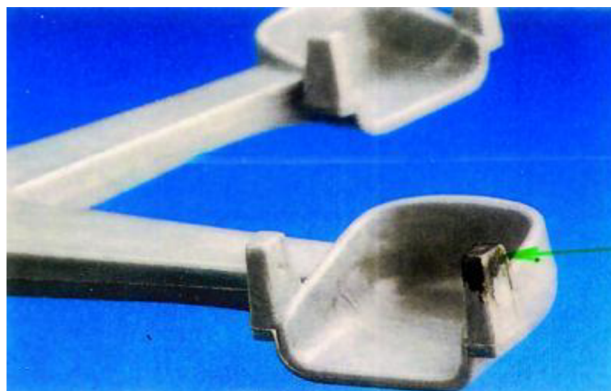
Obr. 31 Dieselefekt [32]
