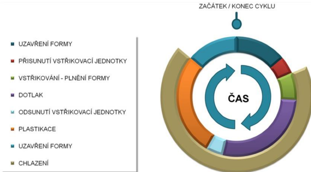
Obr. 23 Vstřikovací cyklus [22]
