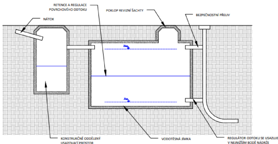
Obrázek 11: Podzemní retenční nádrž (JV PROJEKT HV s.r.o., ©2018)
